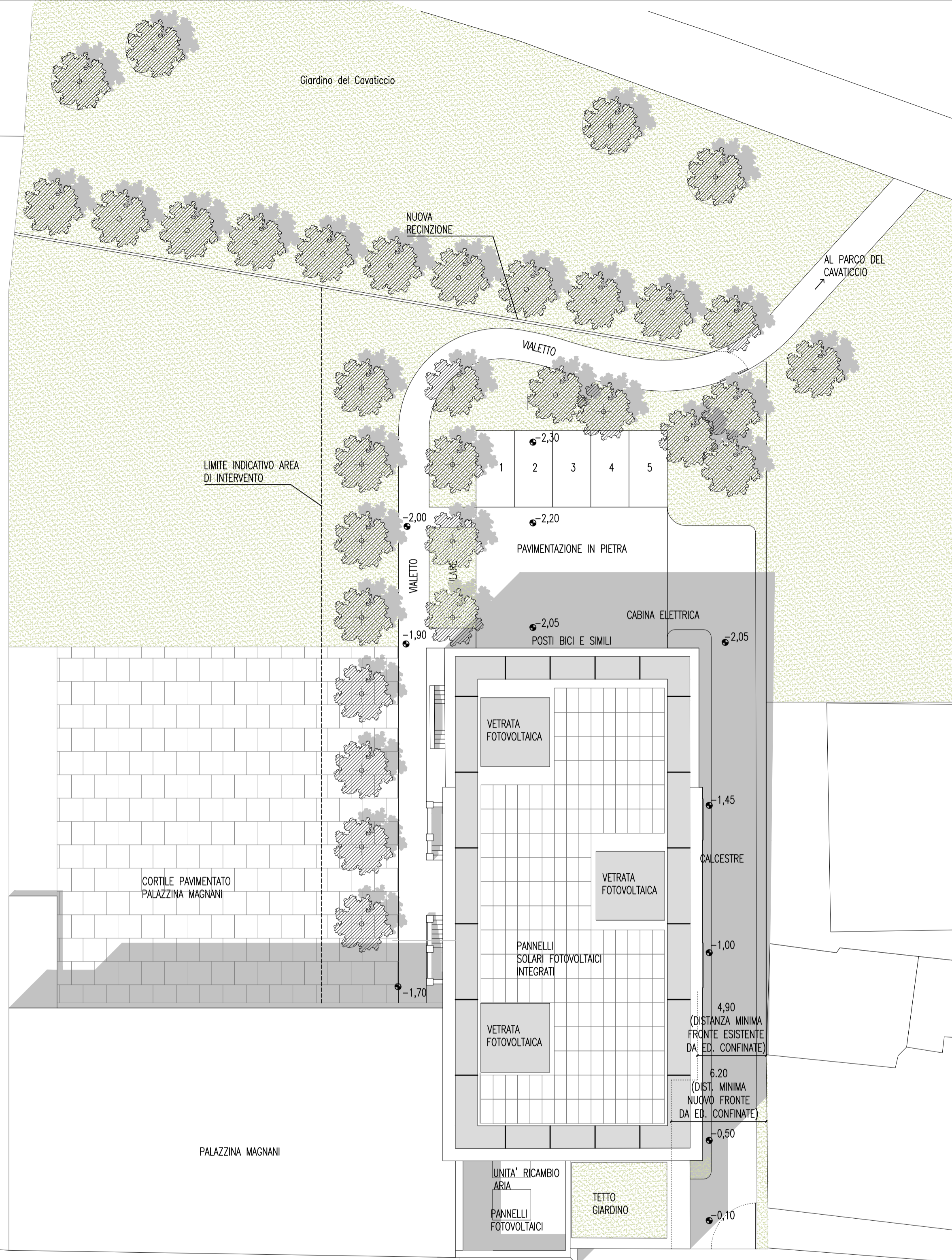
PROGETTO COPERTURE E AREE ESTERNE - SCALA 1:200
