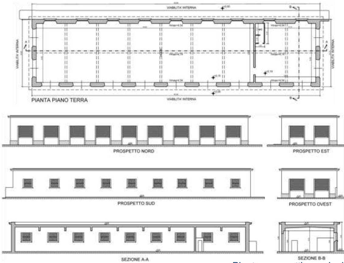
Pianta, prospetti e sezioni
