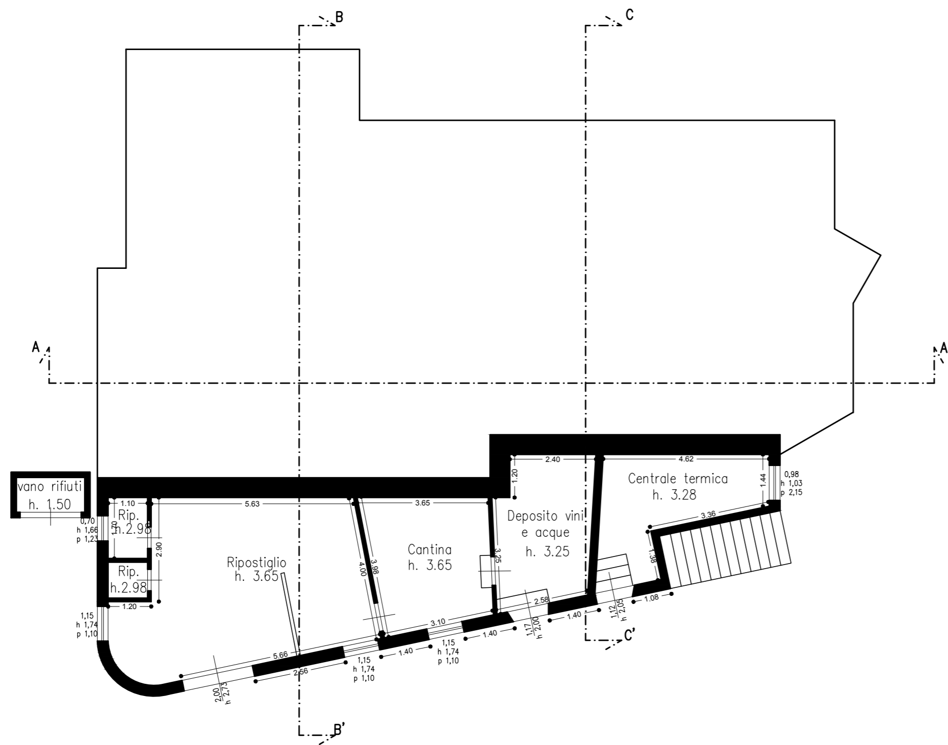
PIANO PRIMO SOTTOSTRADA (SEMINTERRATO)
