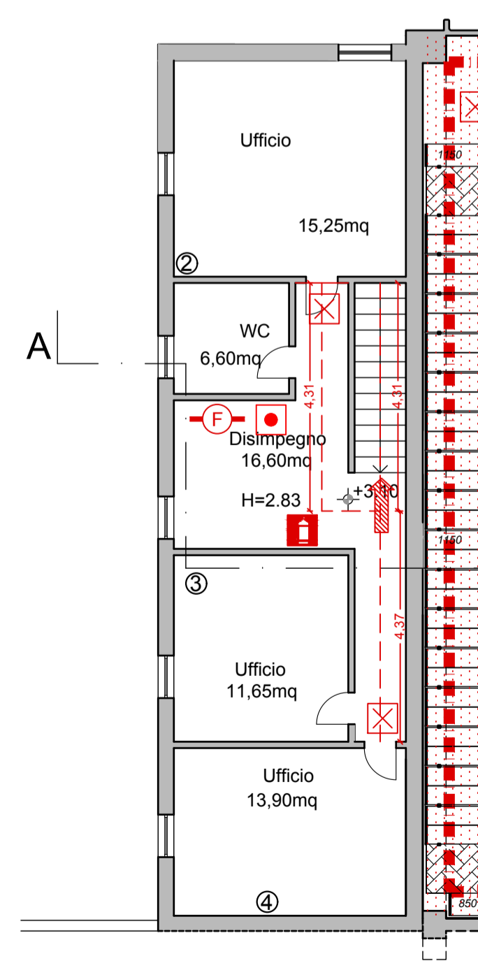
STRALCIO FABBRICATO B - PIANTA PIANO PRIMO
