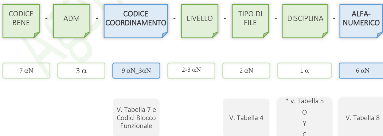
Schema di codifica per i Modelli di Coordinamento Disciplinare, Complessivo, di Synthese e di Blocco Funzionale
