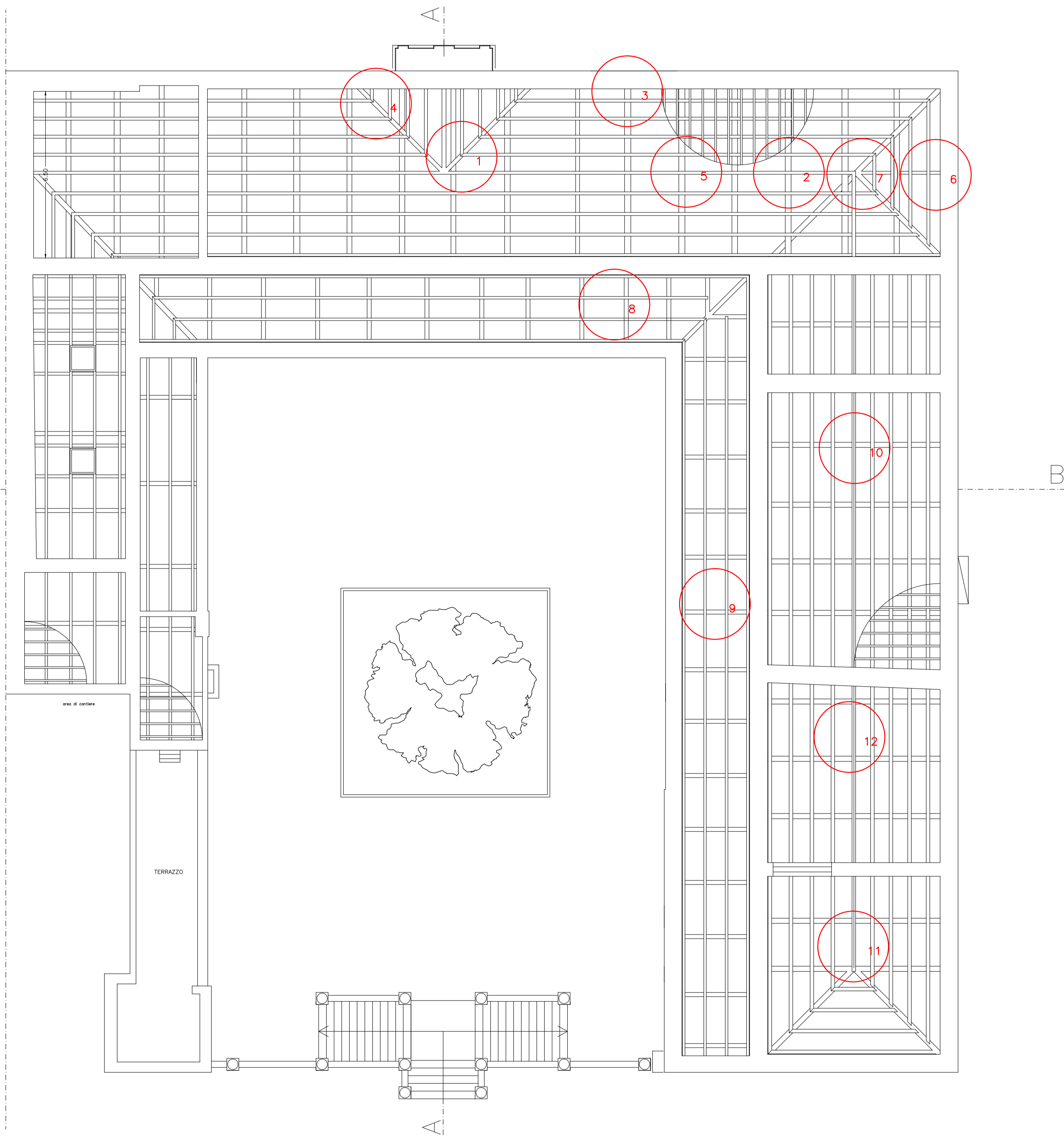
PIANTA DELLE COPERTURE - ORDITURA STRUTTURALE
