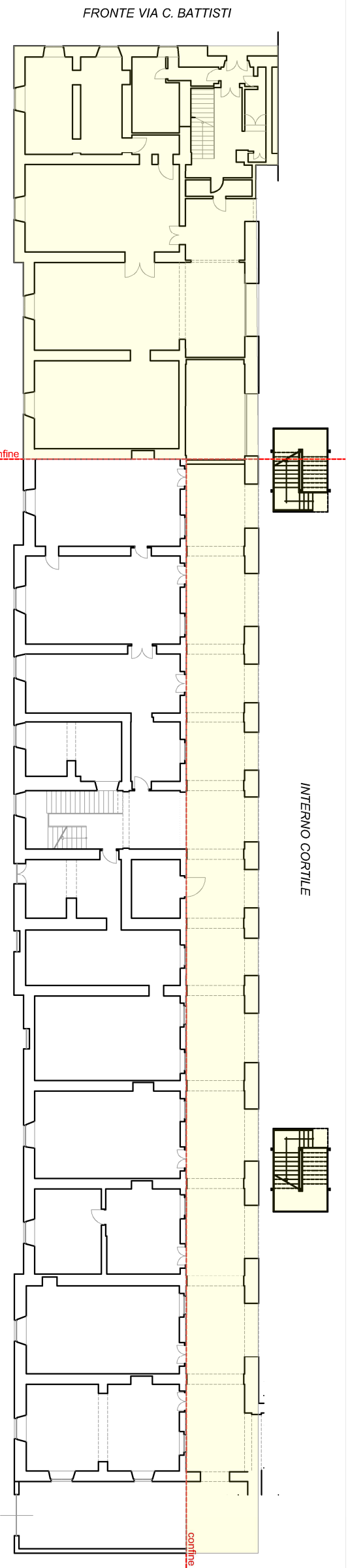
PIANO TERRA SUPERFICE UTILIZZABILE NETTA: 465 mq
