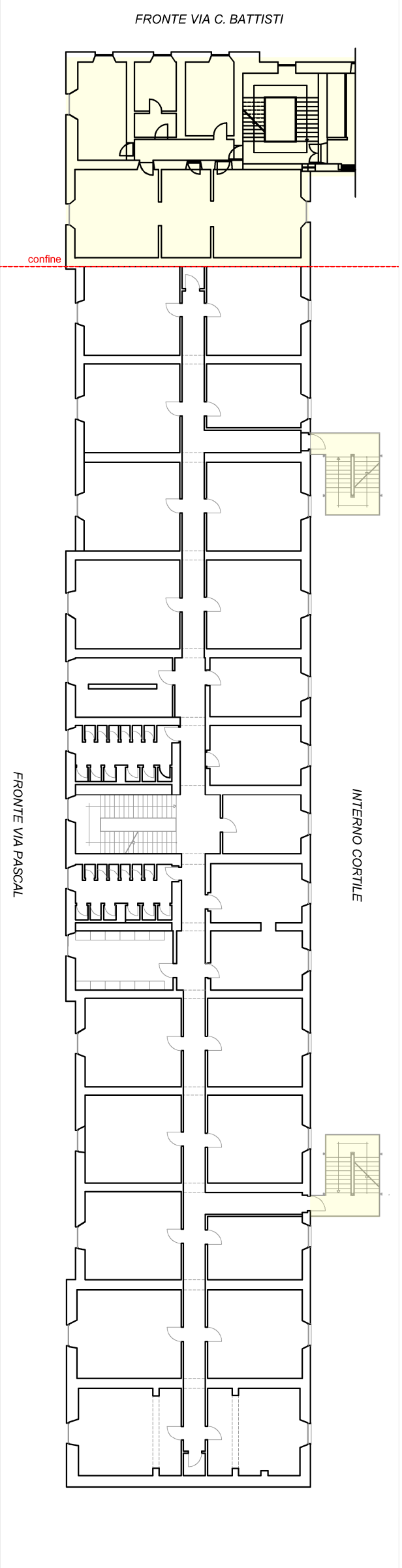
PIANO PRIMO SUPERFICE UTILIZZABILE NETTA: 695 mq
