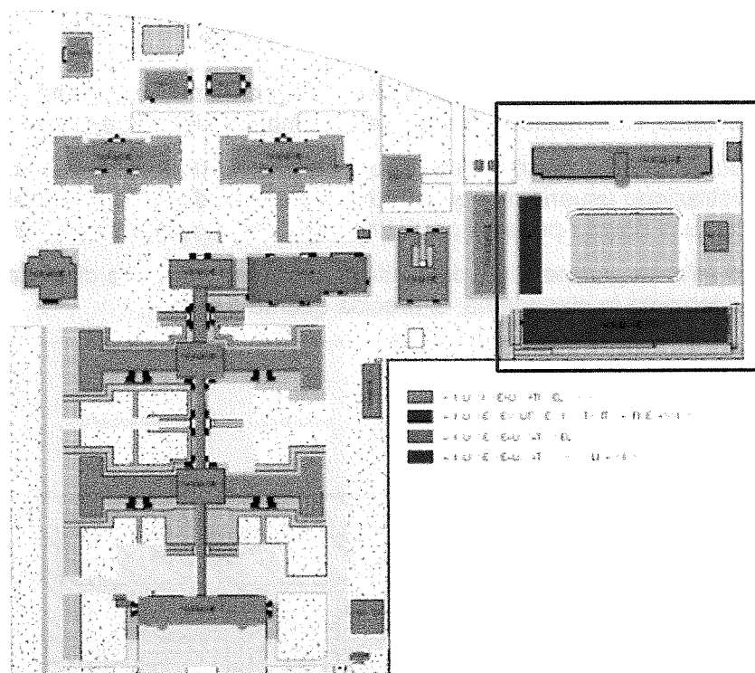
Planimetria con indicazione del perimetro dell'area scoperta oggetto di affidamento della progettazione definitiva
