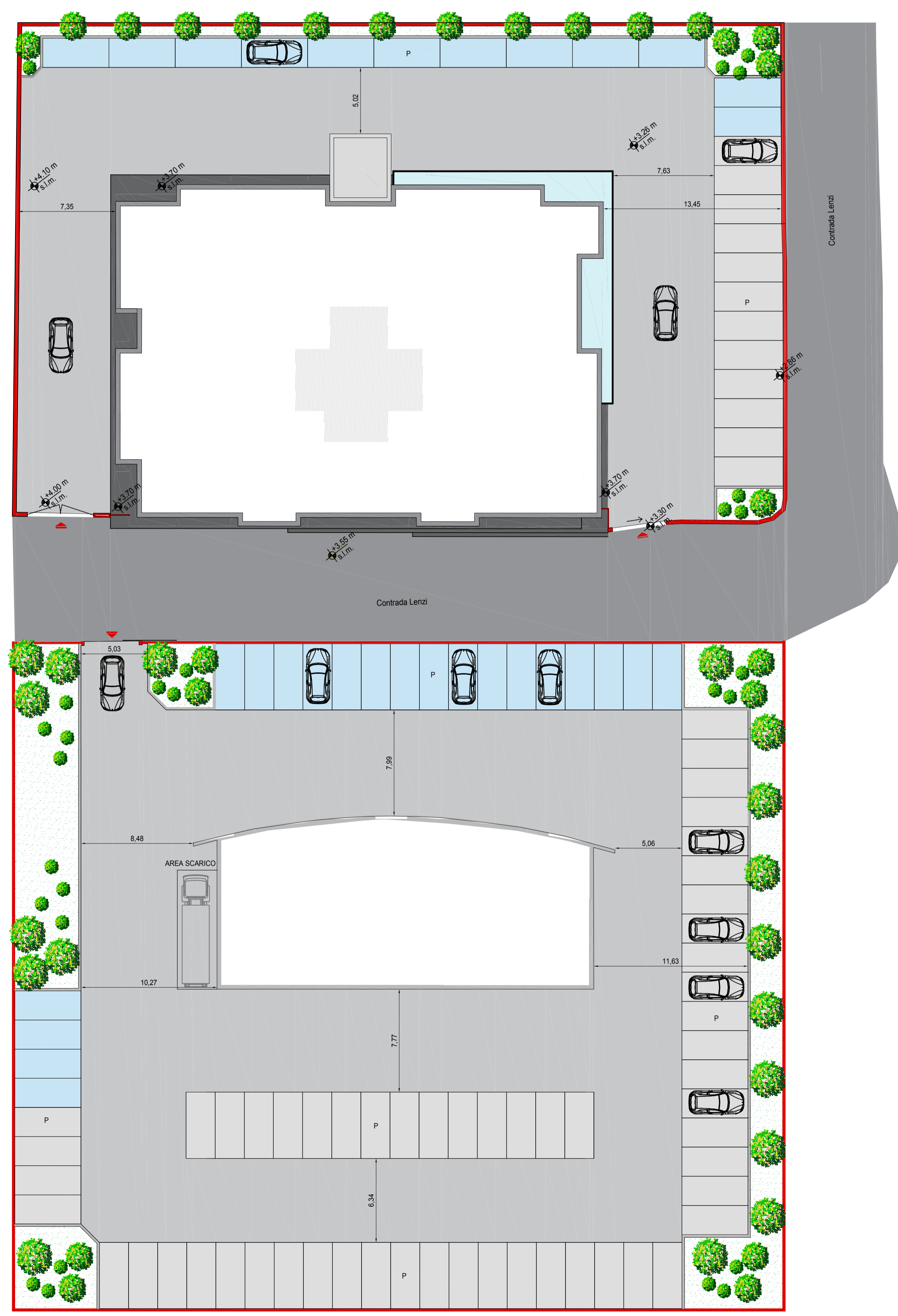
SCHEMA PLANIMETRIA GENERALE (IPOTESI 2) - SCALA 1:200
