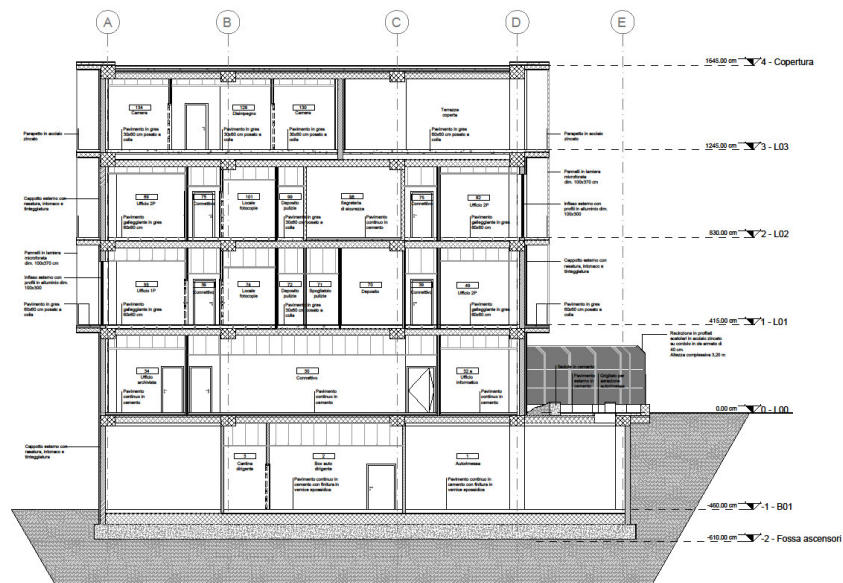
Sezione di progetto
