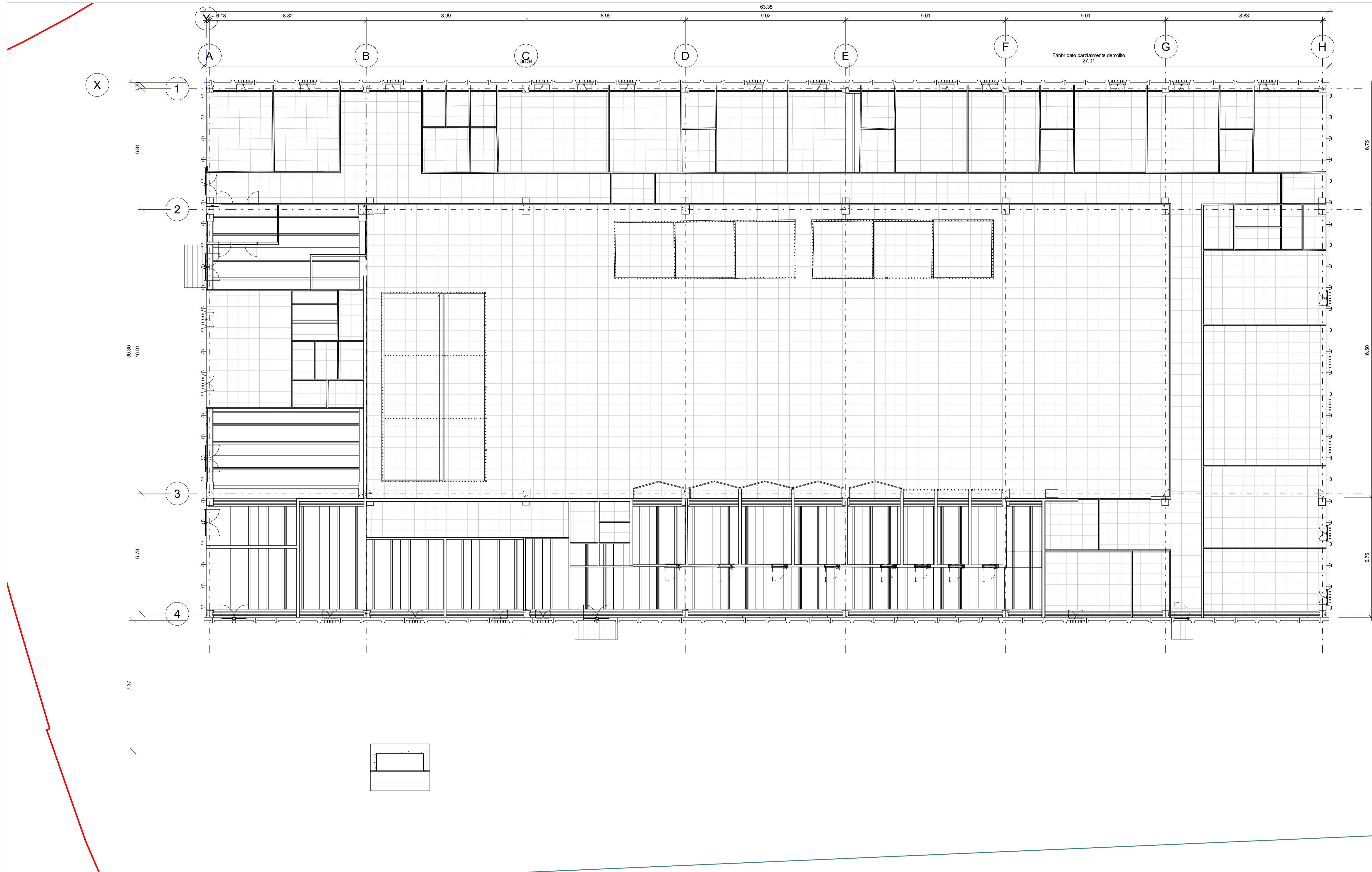
Pianta controsoffitti - Stato di fatto Scala - 1 : 100
