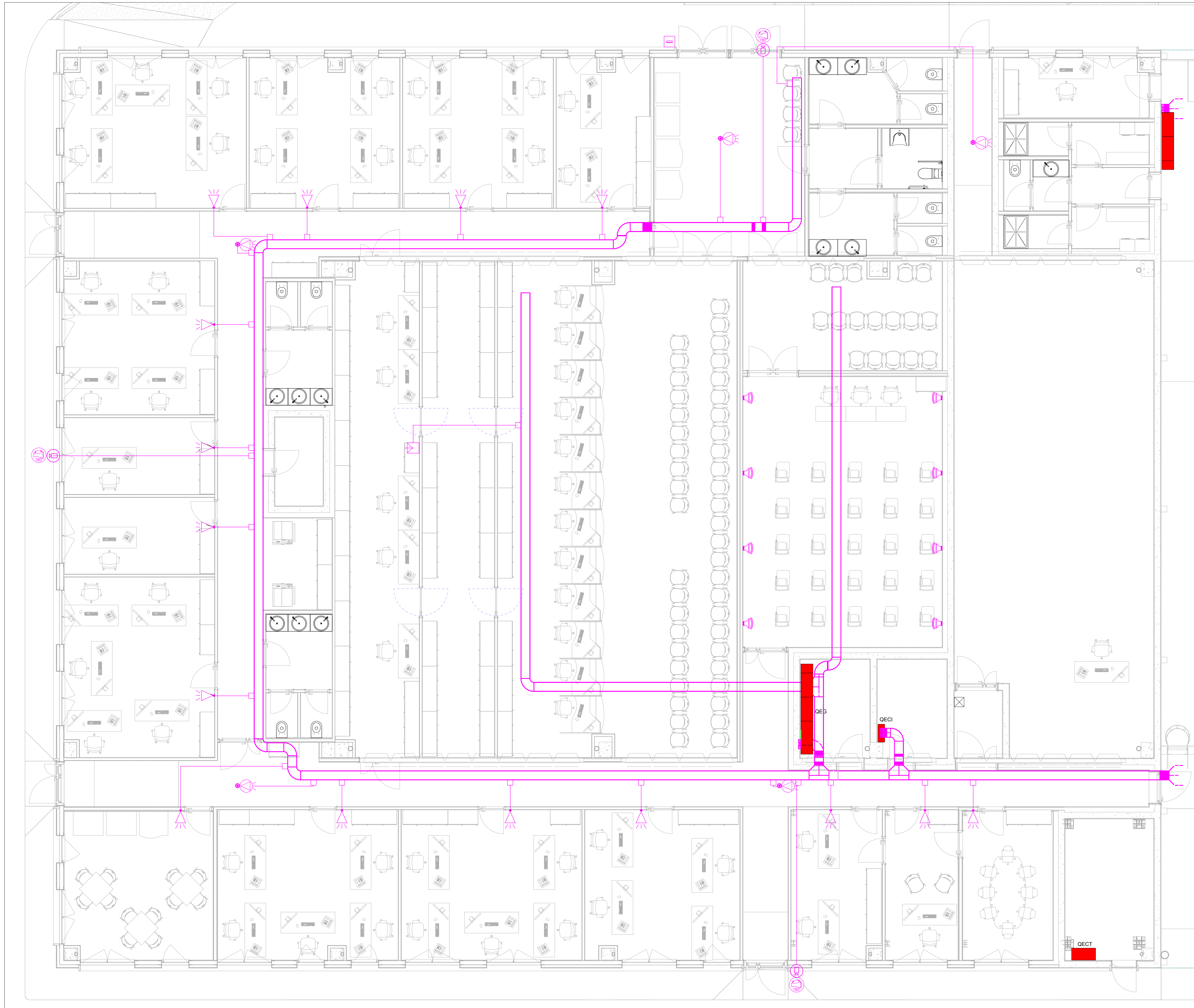
PIANTA UFFICI - ANTINTRUSIONE E VIDEOSORVEGLIANZA SCALA: 1 : 50
