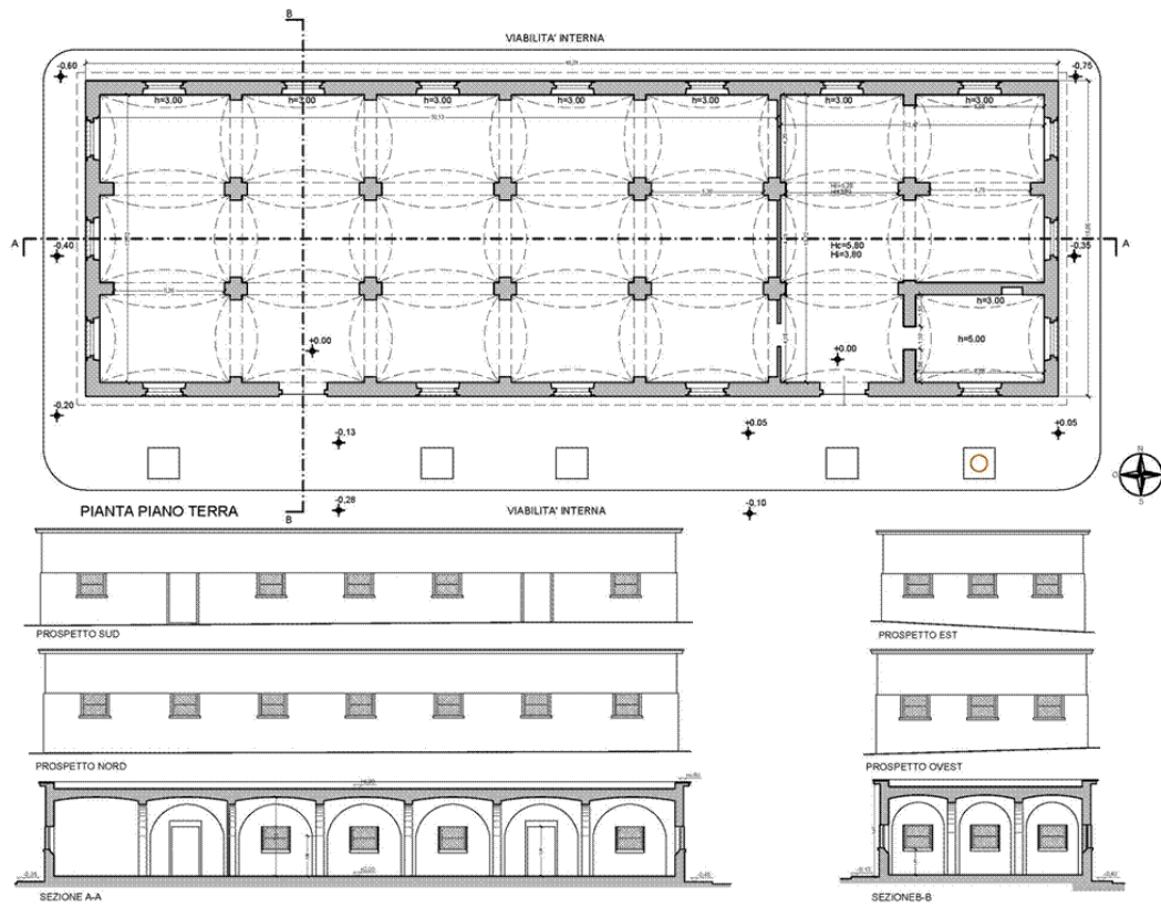
Pianta, prospetti e sezioni
