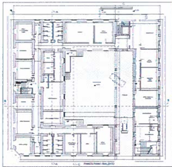
Fabbricato B – pianta piano rialzato, Stato di progetto
