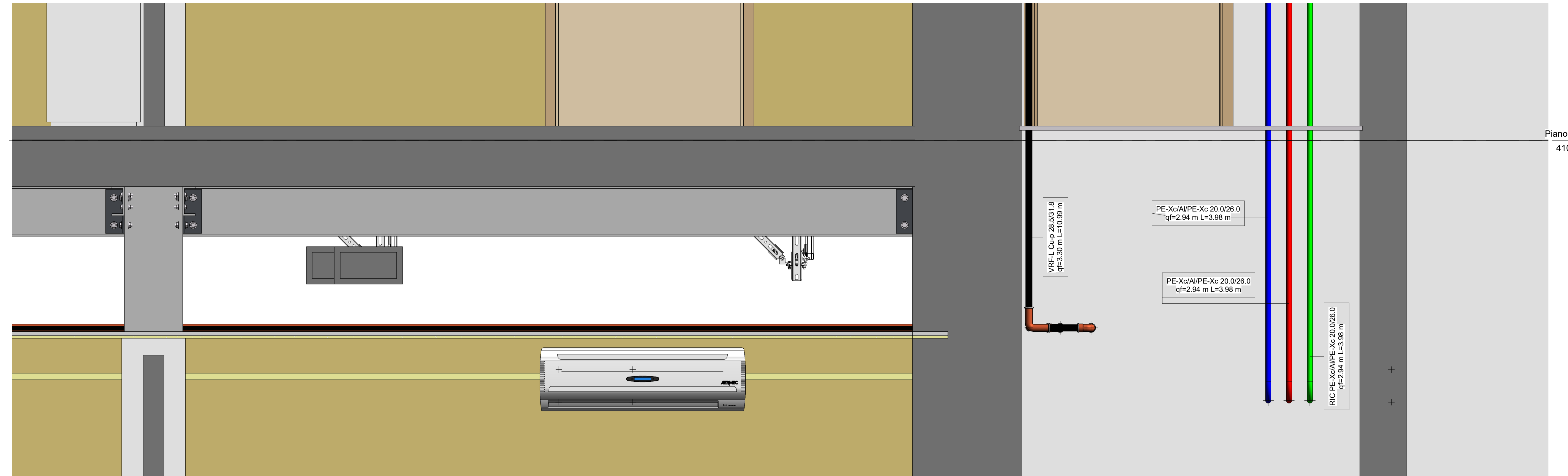
3 Sezione 4 - 02 1 : 10
