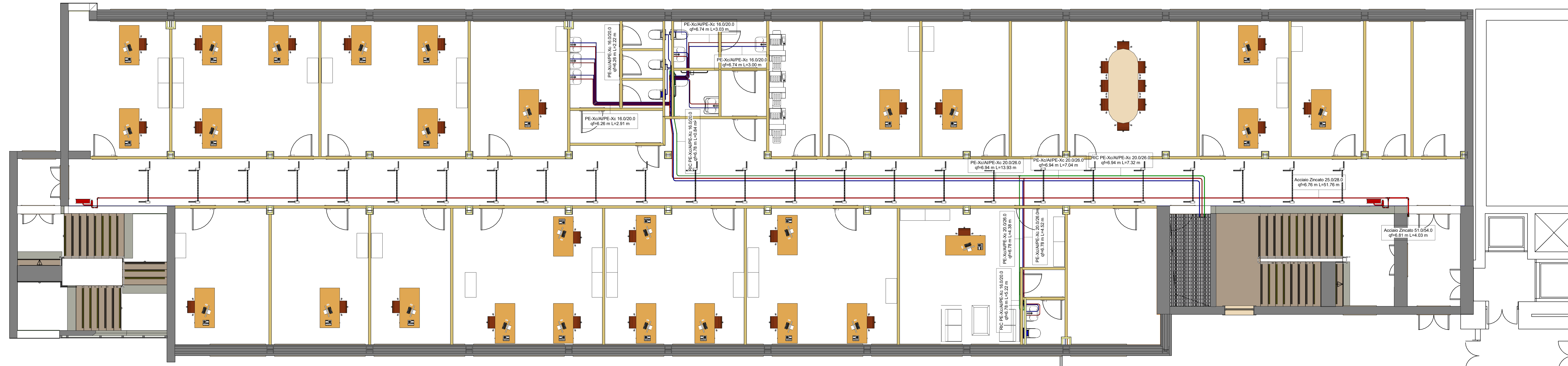
1 Piano Primo - Idrico Sanitario e Antincendio 1:50
