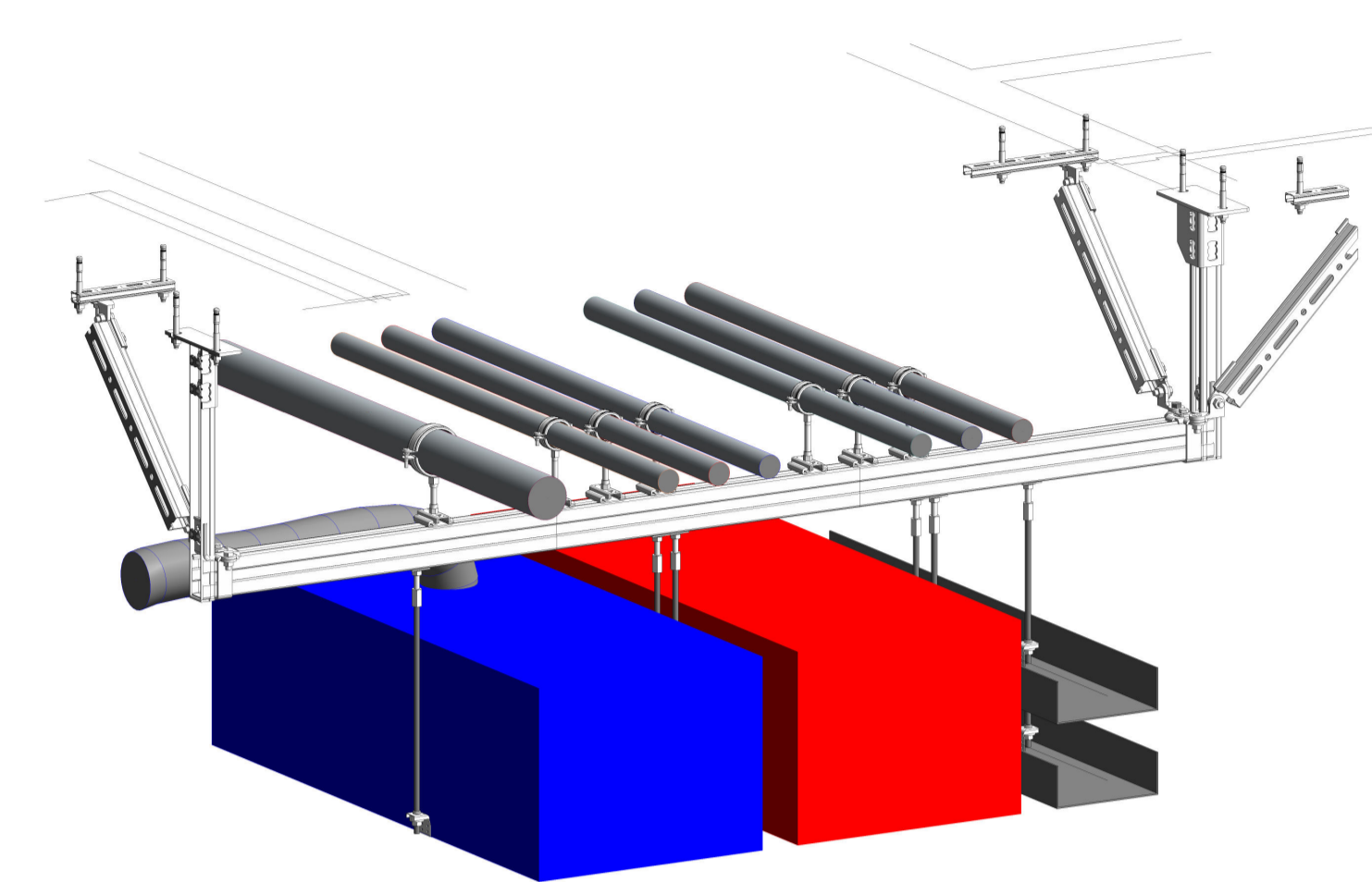
2 staffa 3D - 01 1:1
