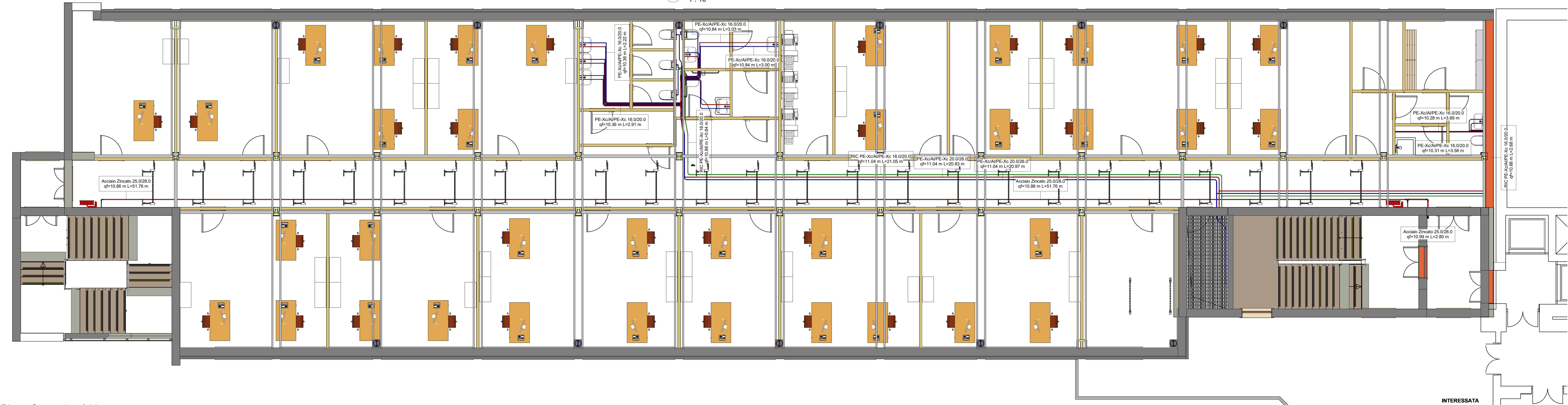
1 Piano Secondo - Idrico Sanitario e Antincendio 1:50
