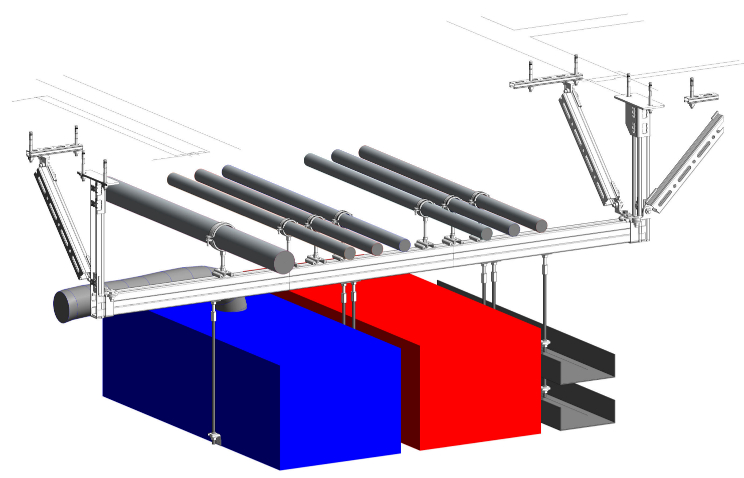
3 staffa 3D - 02 1:1
