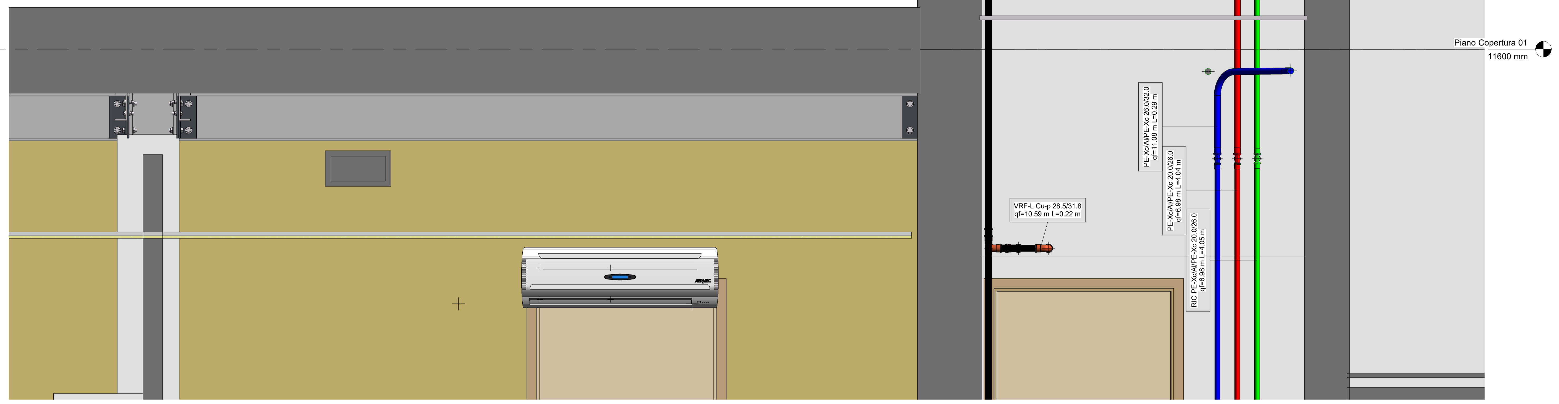
2 Sezione 4 - 03 1:10
