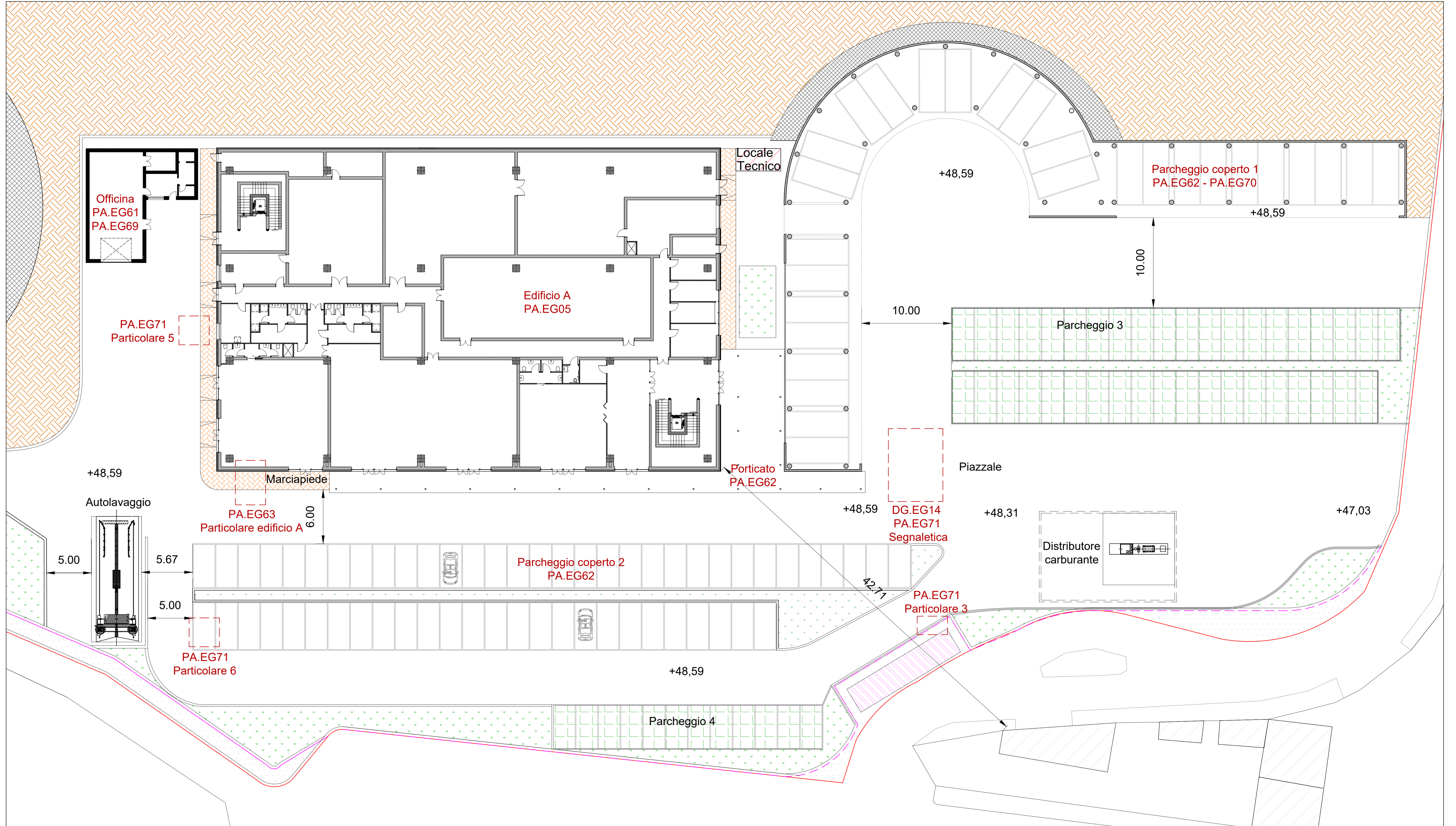
Planimetria generale stato di progetto - Livello piazzale Scala 1:200
