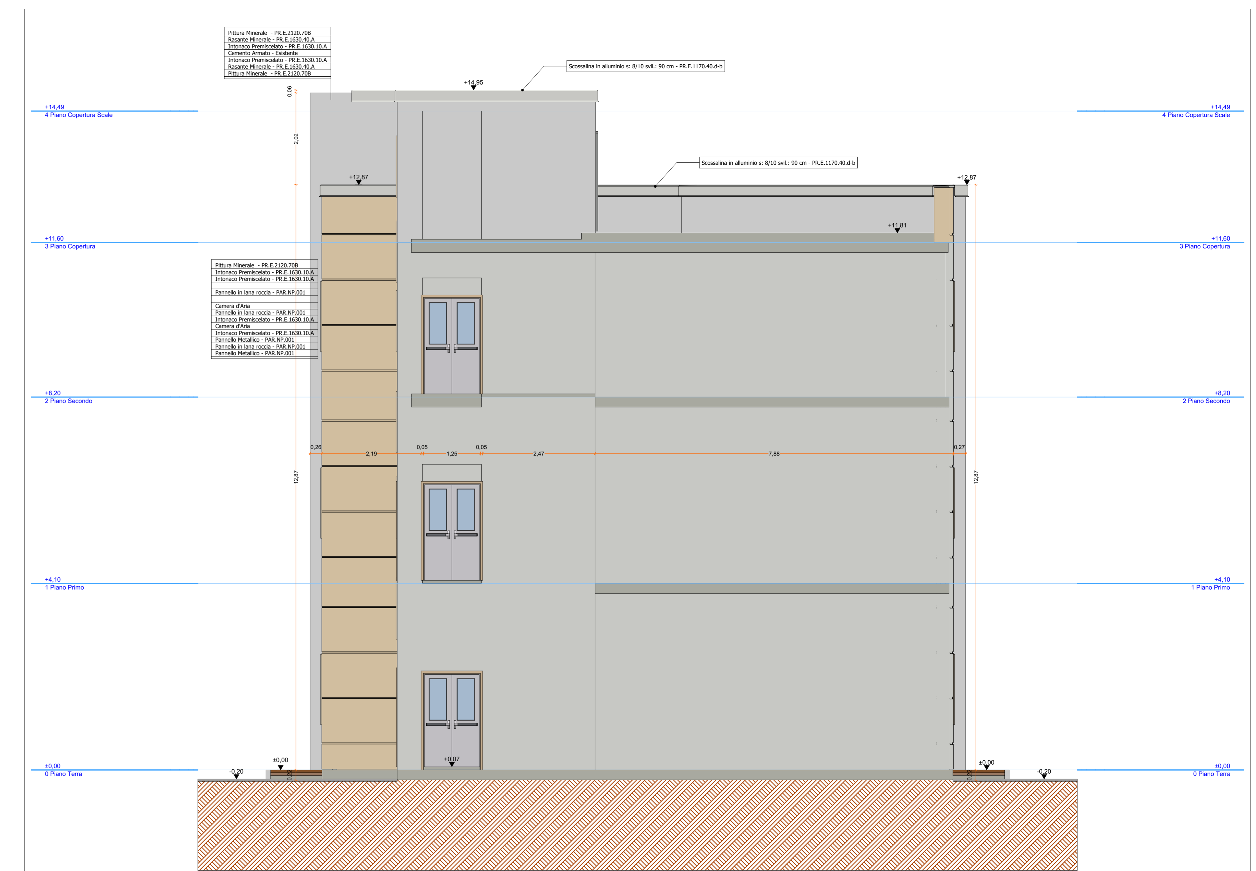
Prospetto Sud 1:50
