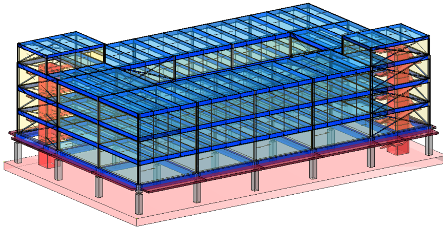
Vista del Modello Estruso 3D
