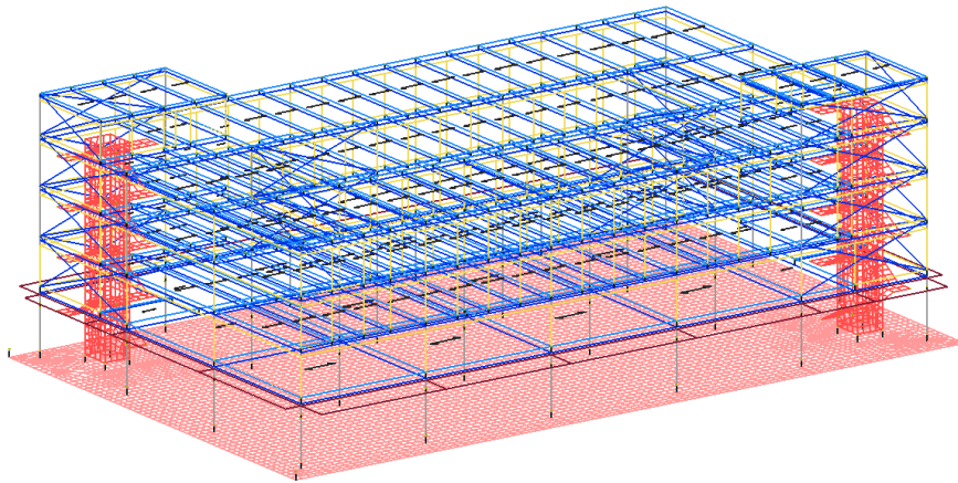
Vista del Modello FEM 3D
