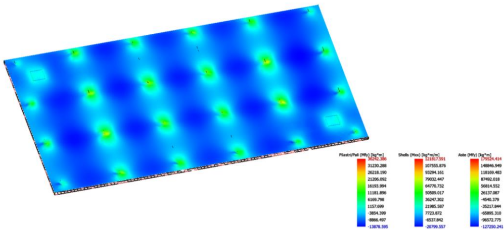
Diagramma sollecitazioni Mxx – SISMAY1_SLV
