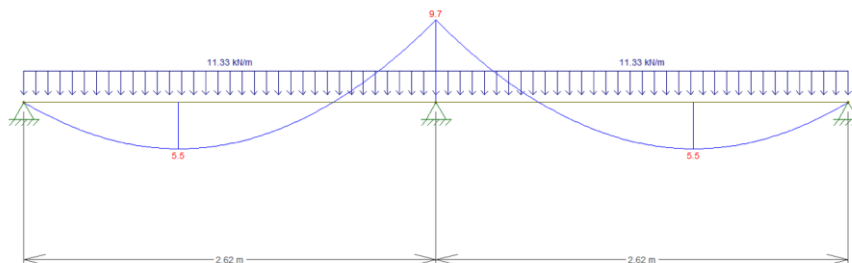
Sollecitazione Flettente
