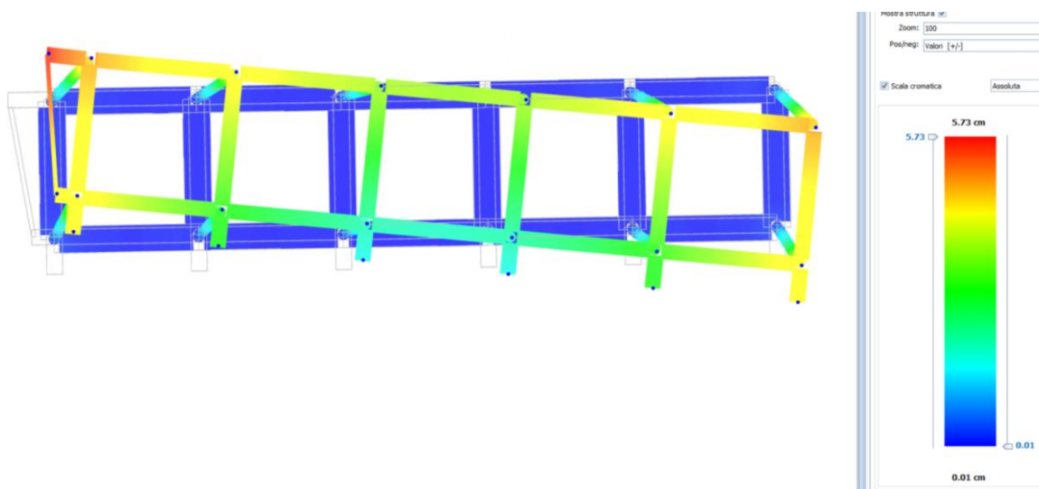
Schema spostamenti blocco n.1 dir. X
