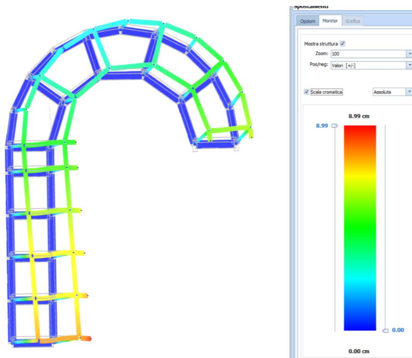
Schema spostamenti blocco n.2 dir. X
