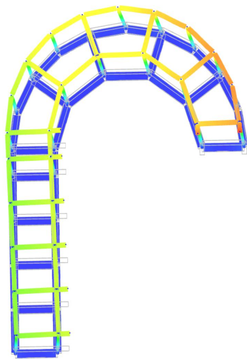
Schema spostamenti blocco n.2 dir.Y
