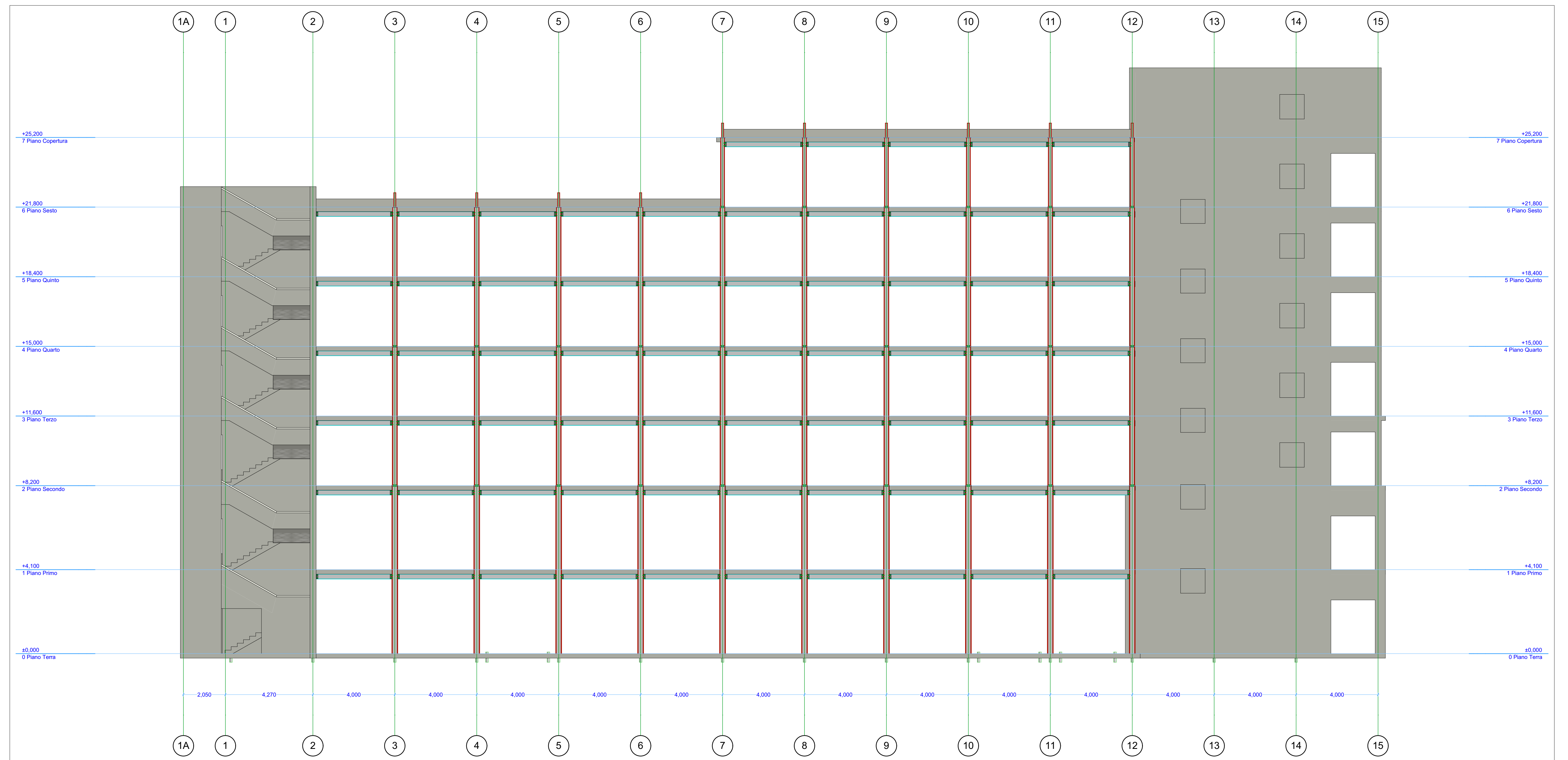
2 Prospetto Ovest 1:100
