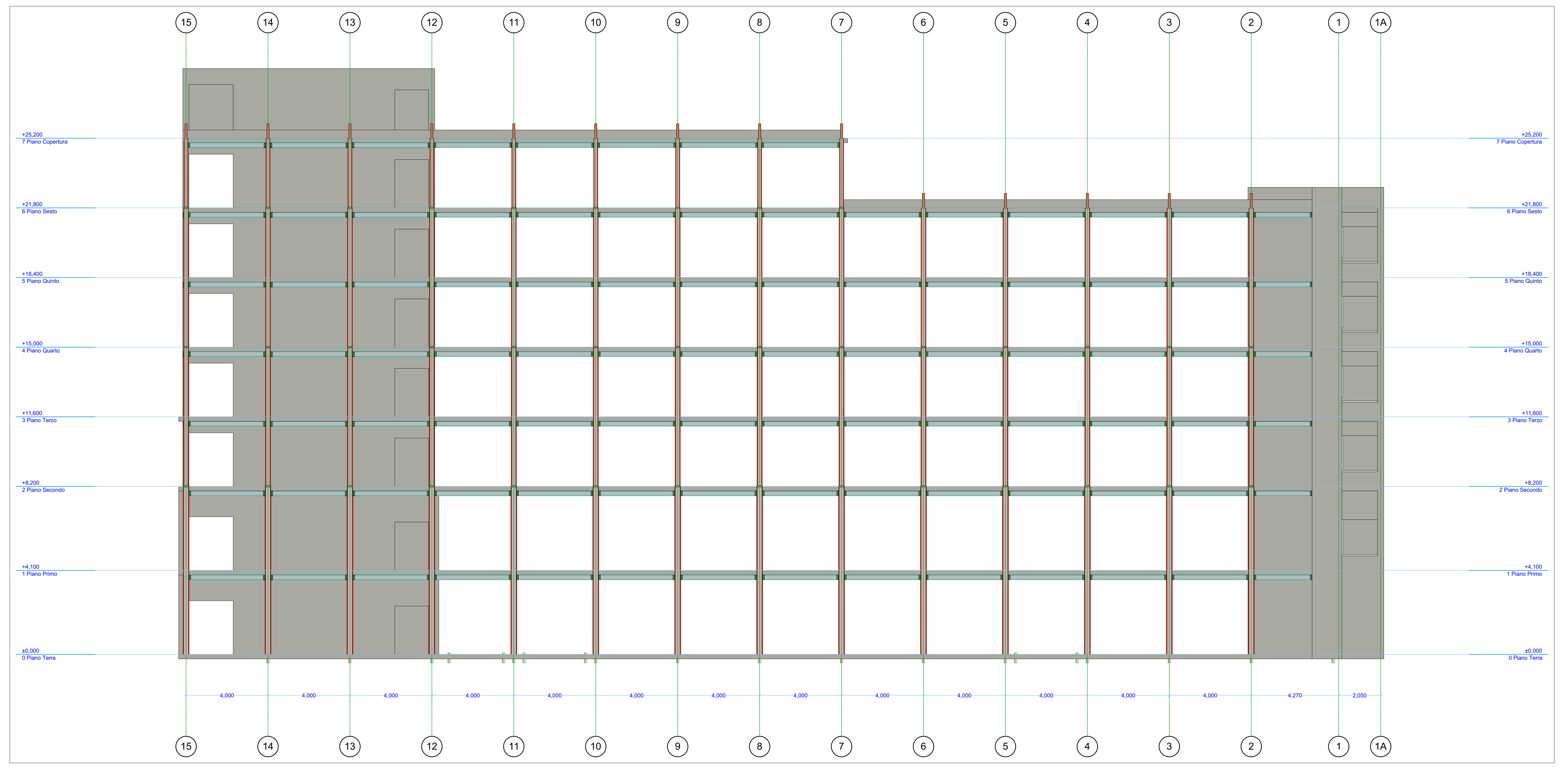
1 Prospetto Est 1:100
