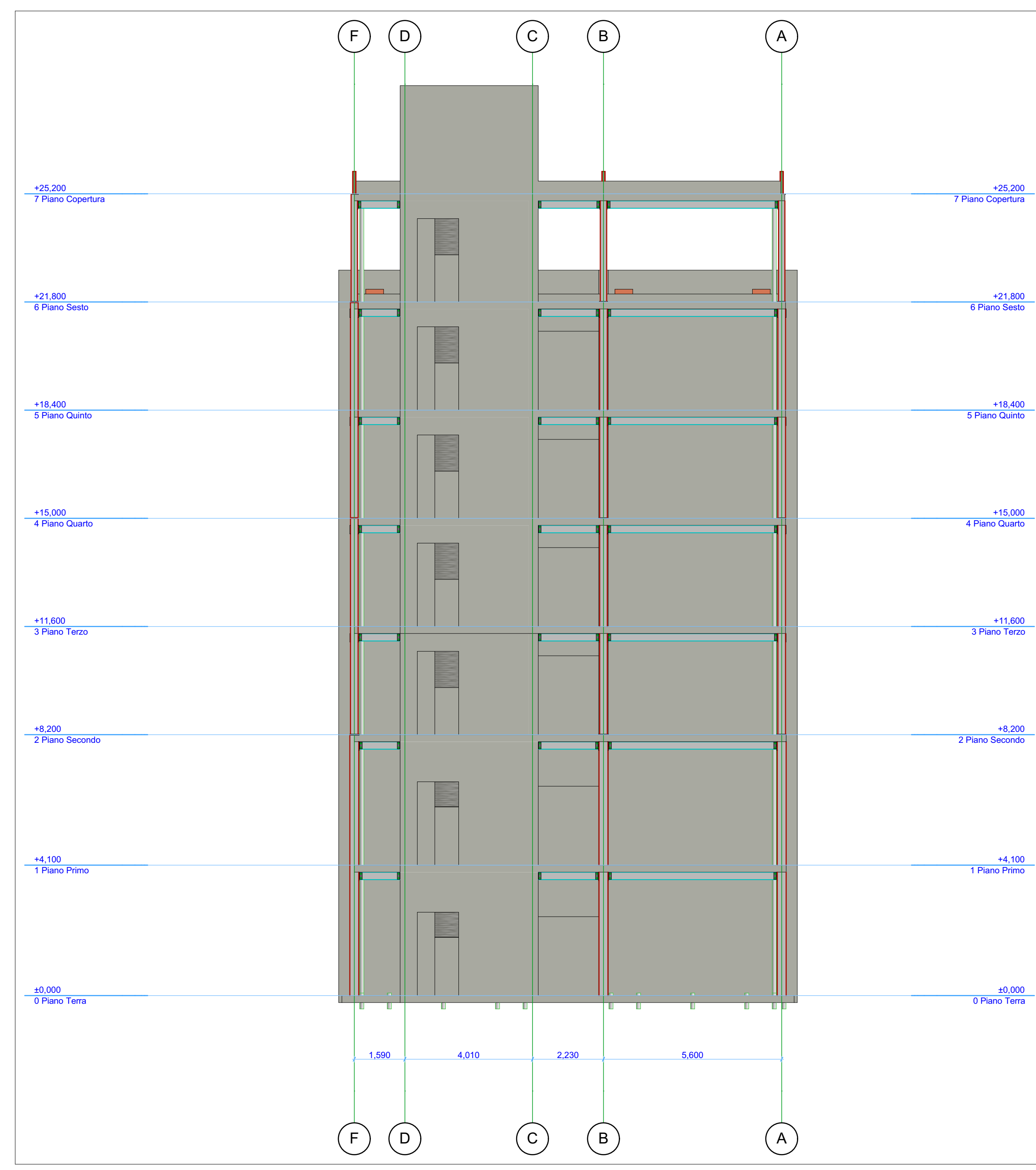
3 Alzato Sud 1:100
