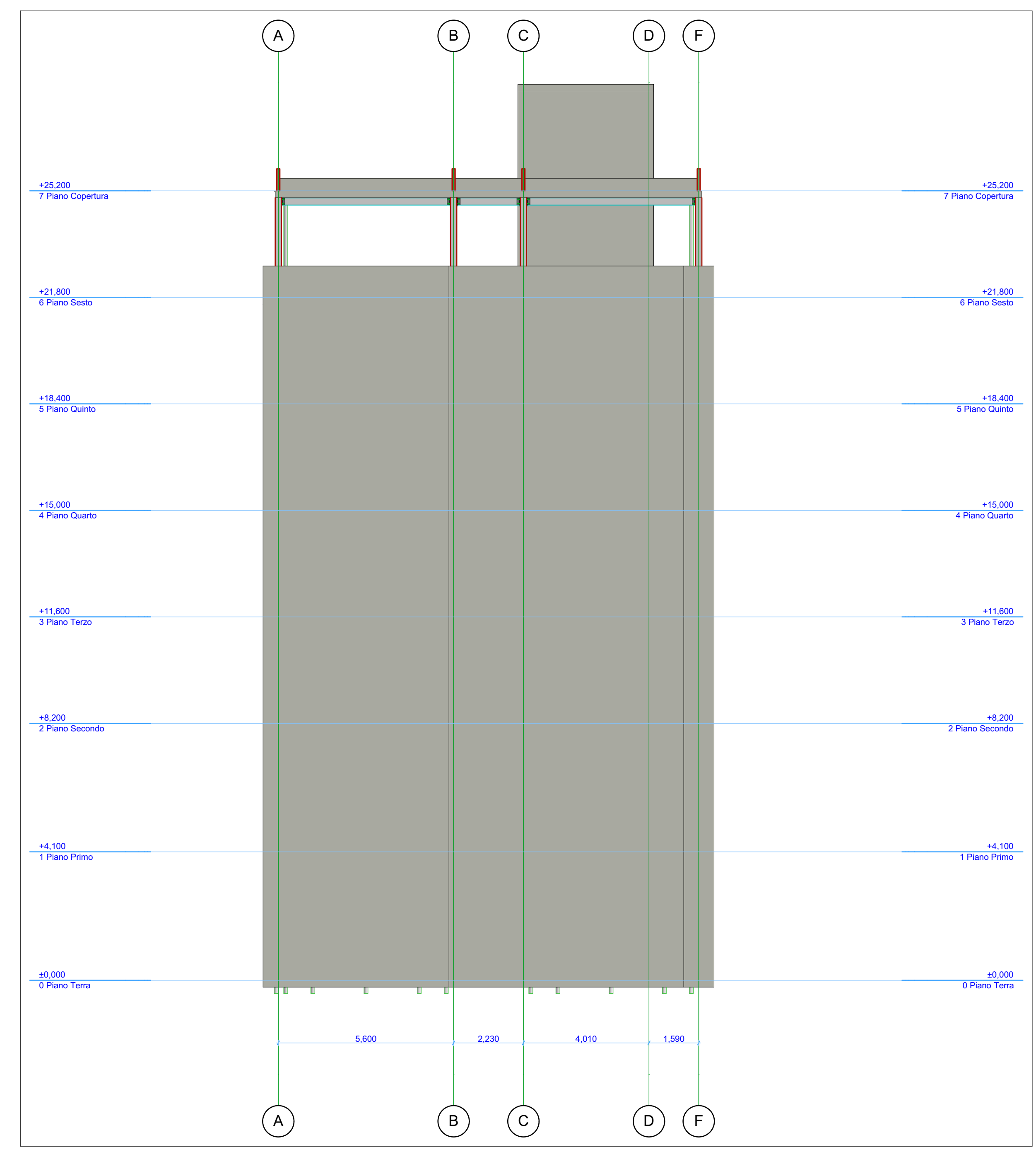
4 Alzato Nord 1:100
