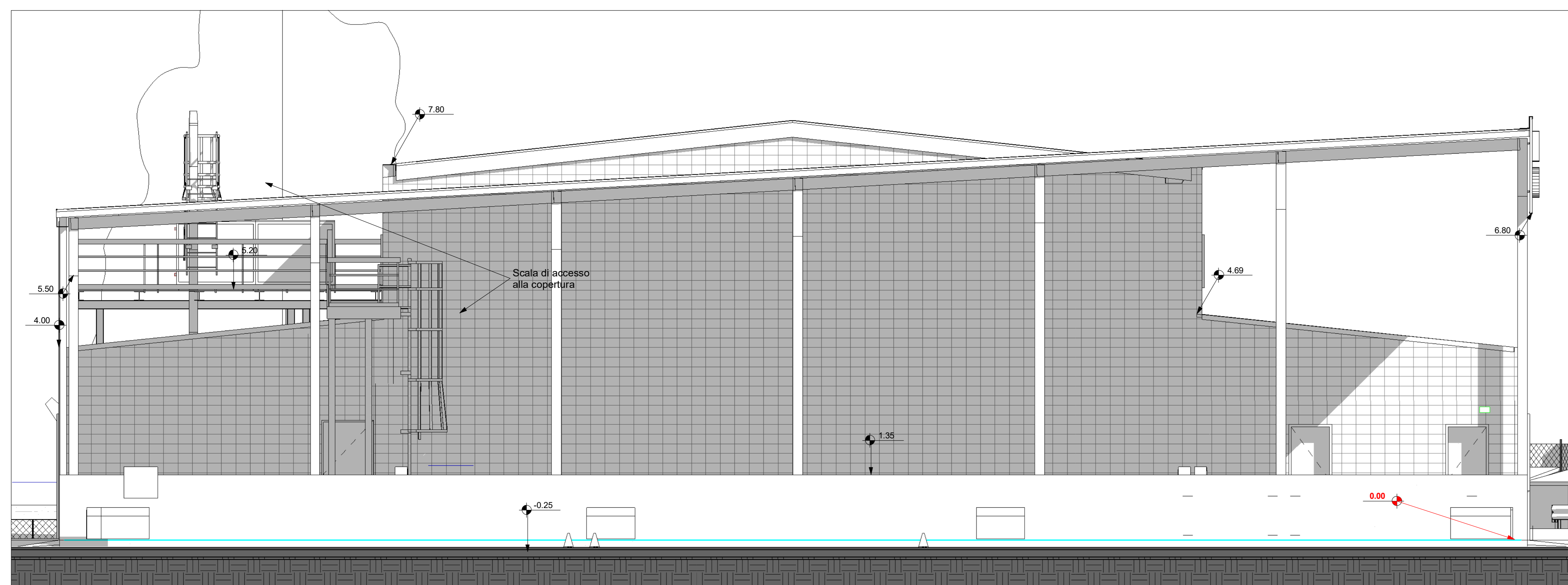
Prospetto Est Scala: 1:50
