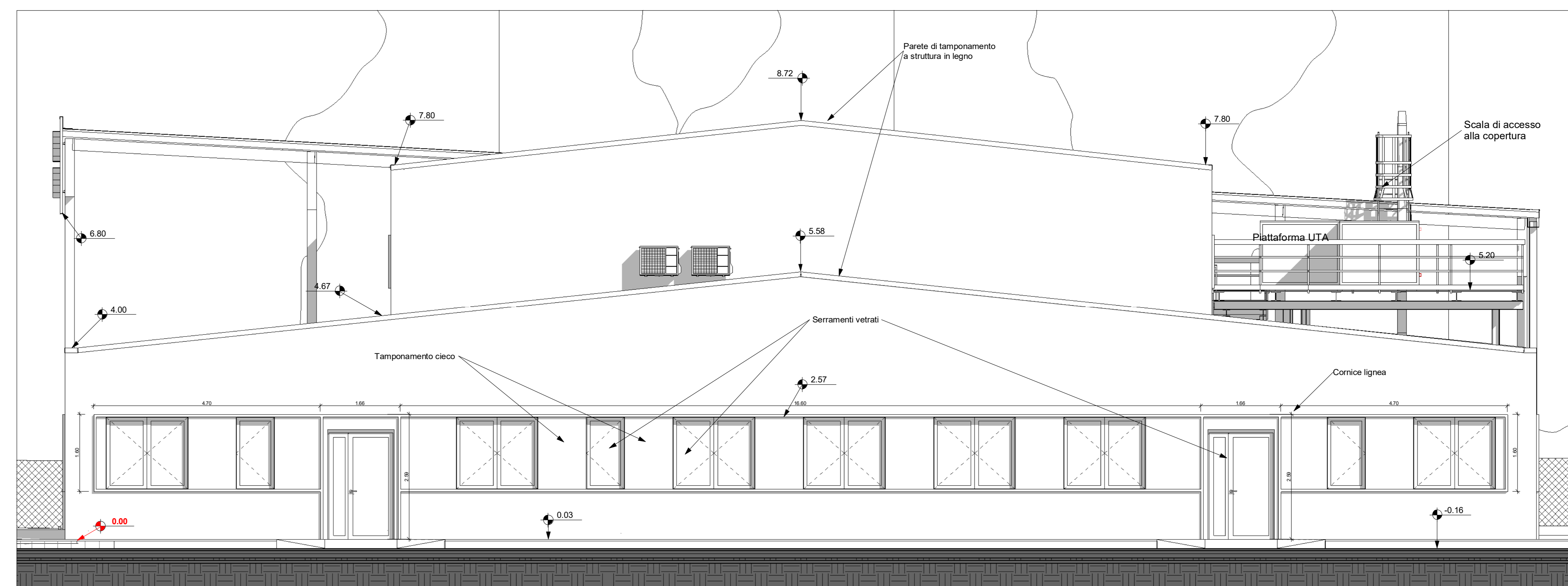
Prospetto Ovest Scala: 1:50
