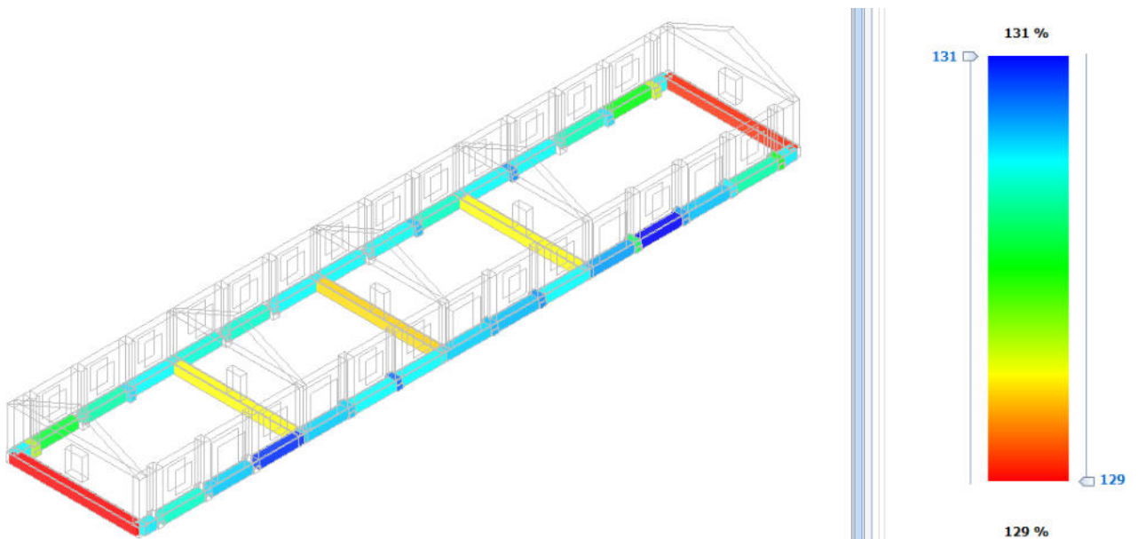
Figura 6 - Accelerazione sismica di collasso – Carico terreno
