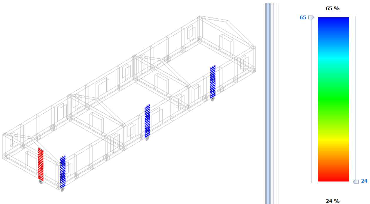
Figura 5 - Accelerazione sismica di collasso – Cinematismo SLV PGA
