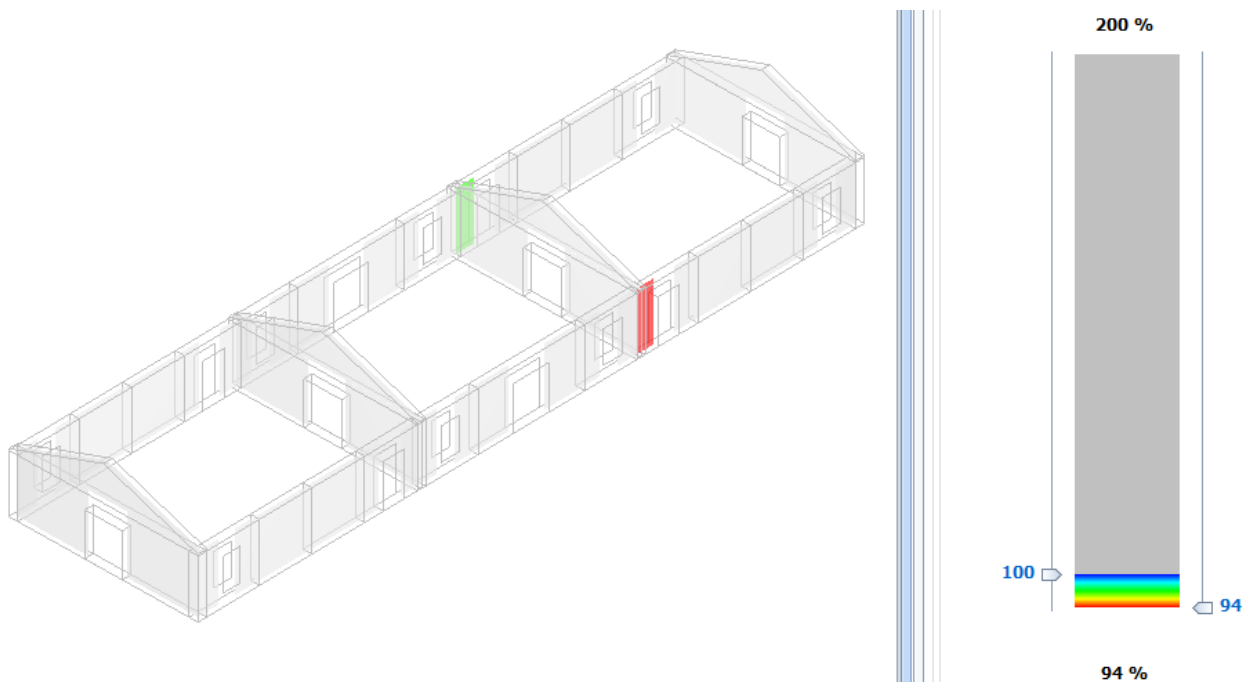
Figura 1 - Accelerazione sismica di collasso – Pressoflessione nel piano
