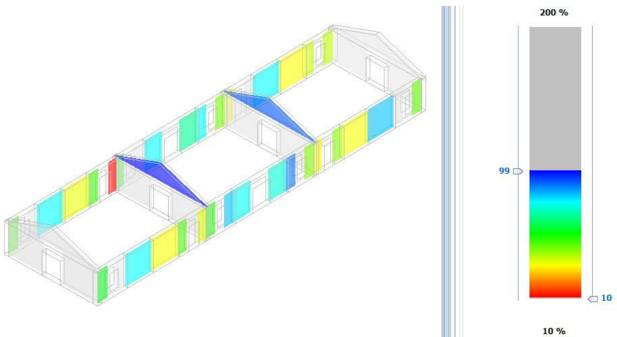
Figura 2 - Accelerazione sismica di collasso – Pressoflessione fuori piano
