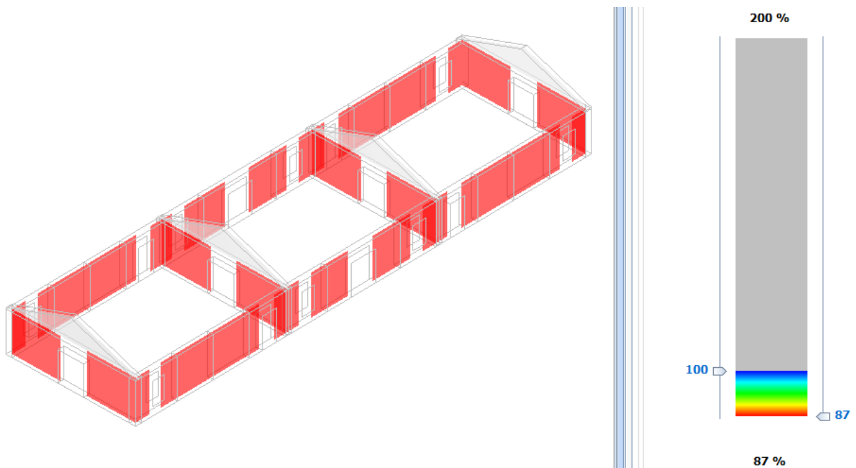
Figura 4 - Accelerazione sismica di collasso – Deformazione ultima
