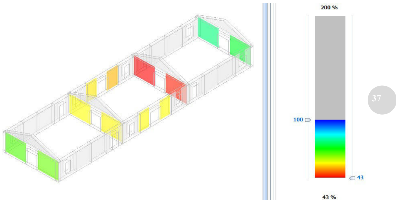
Figura 3 - Accelerazione sismica di collasso – Taglio nel piano
