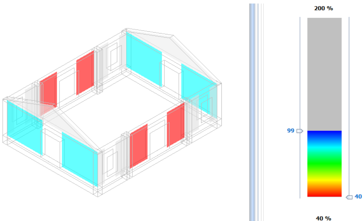
Figura 3 - Accelerazione sismica di collasso – Taglio nel piano
