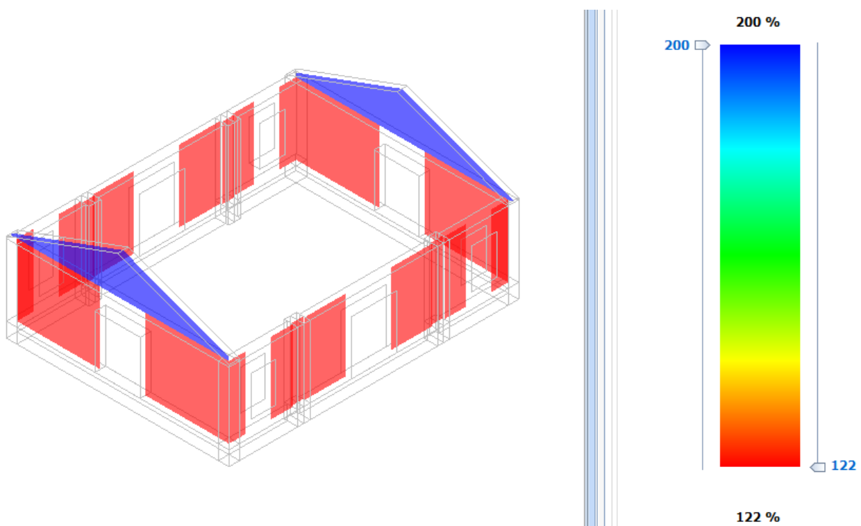
Figura 4 - Accelerazione sismica di collasso – Deformazione ultima
