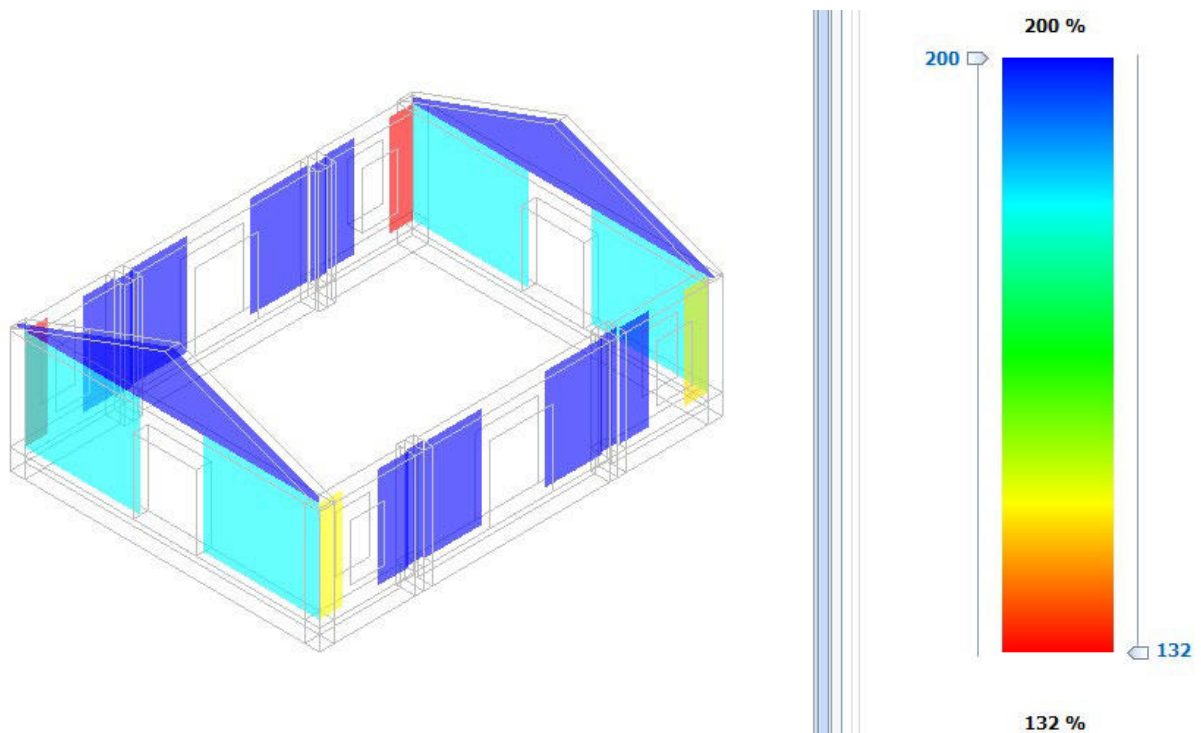
Figura 1 - Accelerazione sismica di collasso – Pressoflessione nel piano
