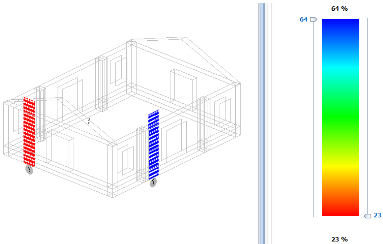
Figura 5 - Accelerazione sismica di collasso – Cinematismo SLV PGA
