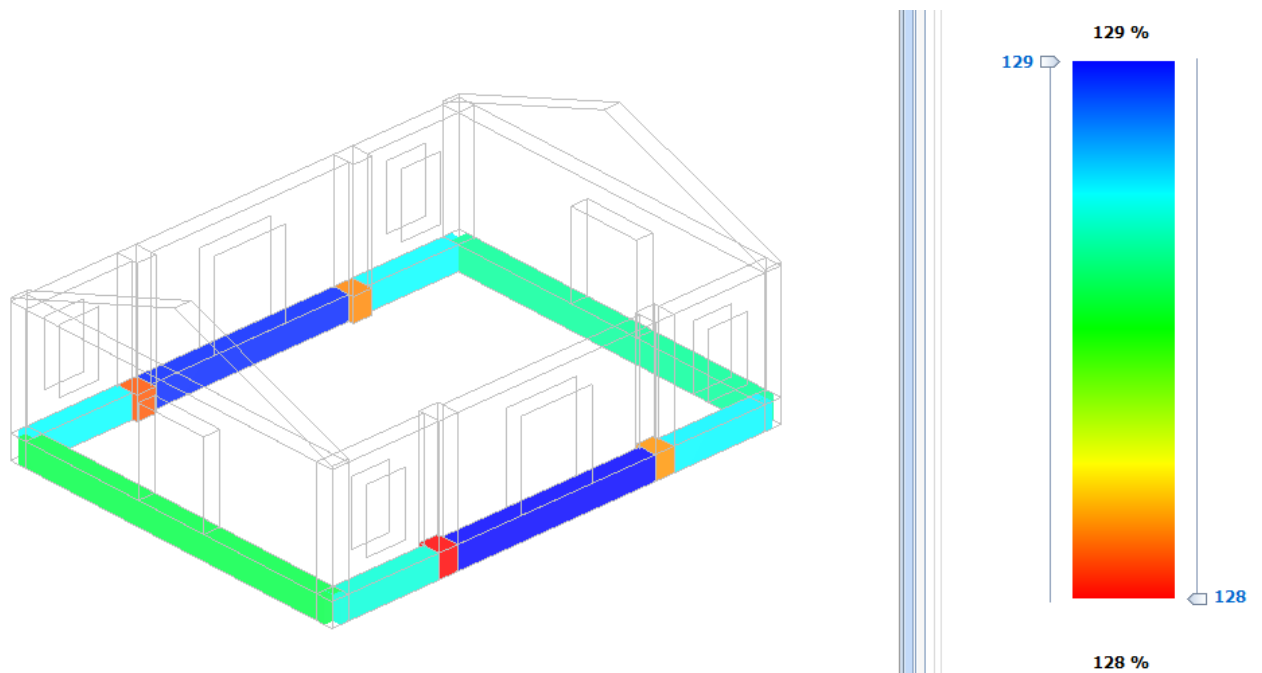
Figura 6 - Accelerazione sismica di collasso – Carico terreno
