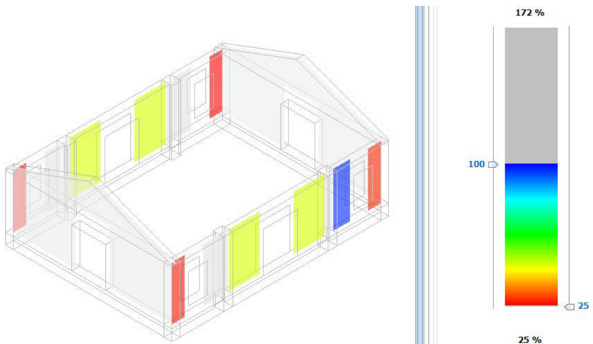
Figura 2 - Accelerazione sismica di collasso – Pressoflessione fuori casa
