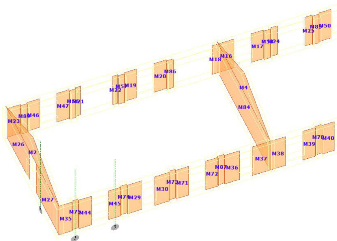
Figura 2 – Numerazione maschi murari
