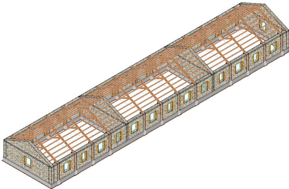
Figura 1 – Modello FEM
