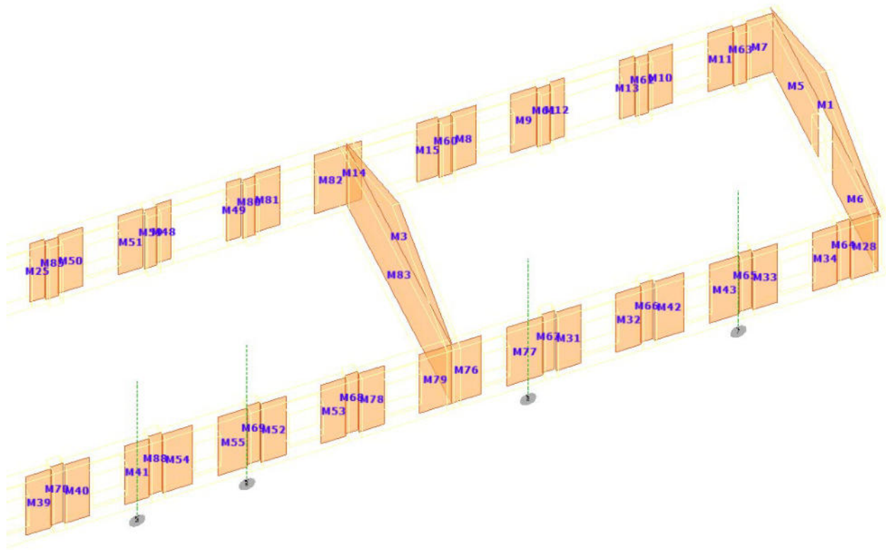
Figura 3 – Numerazione maschi murari
