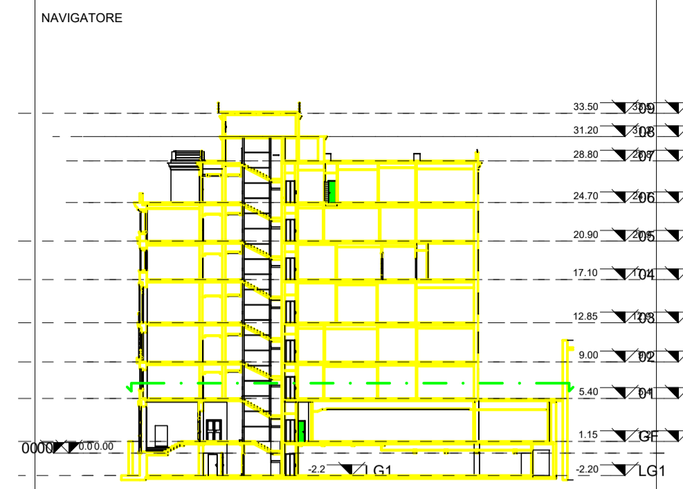
Piano di sezione +1.50m
