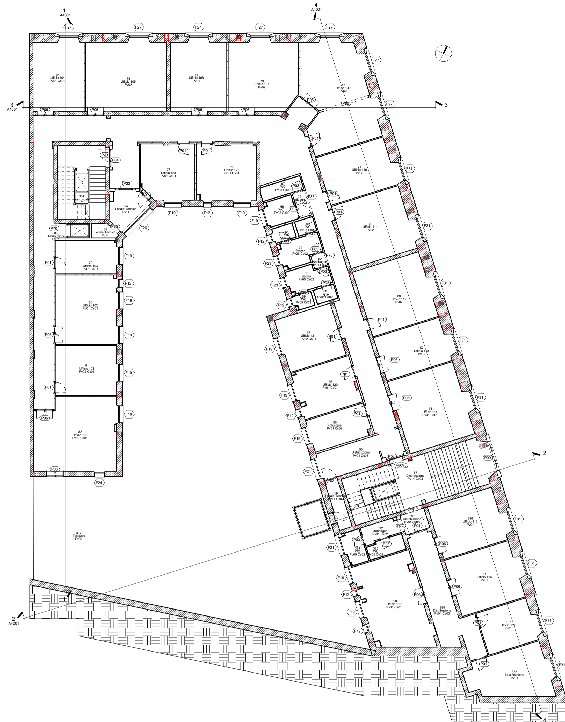
A_01_Funzionale Scala 1:100
