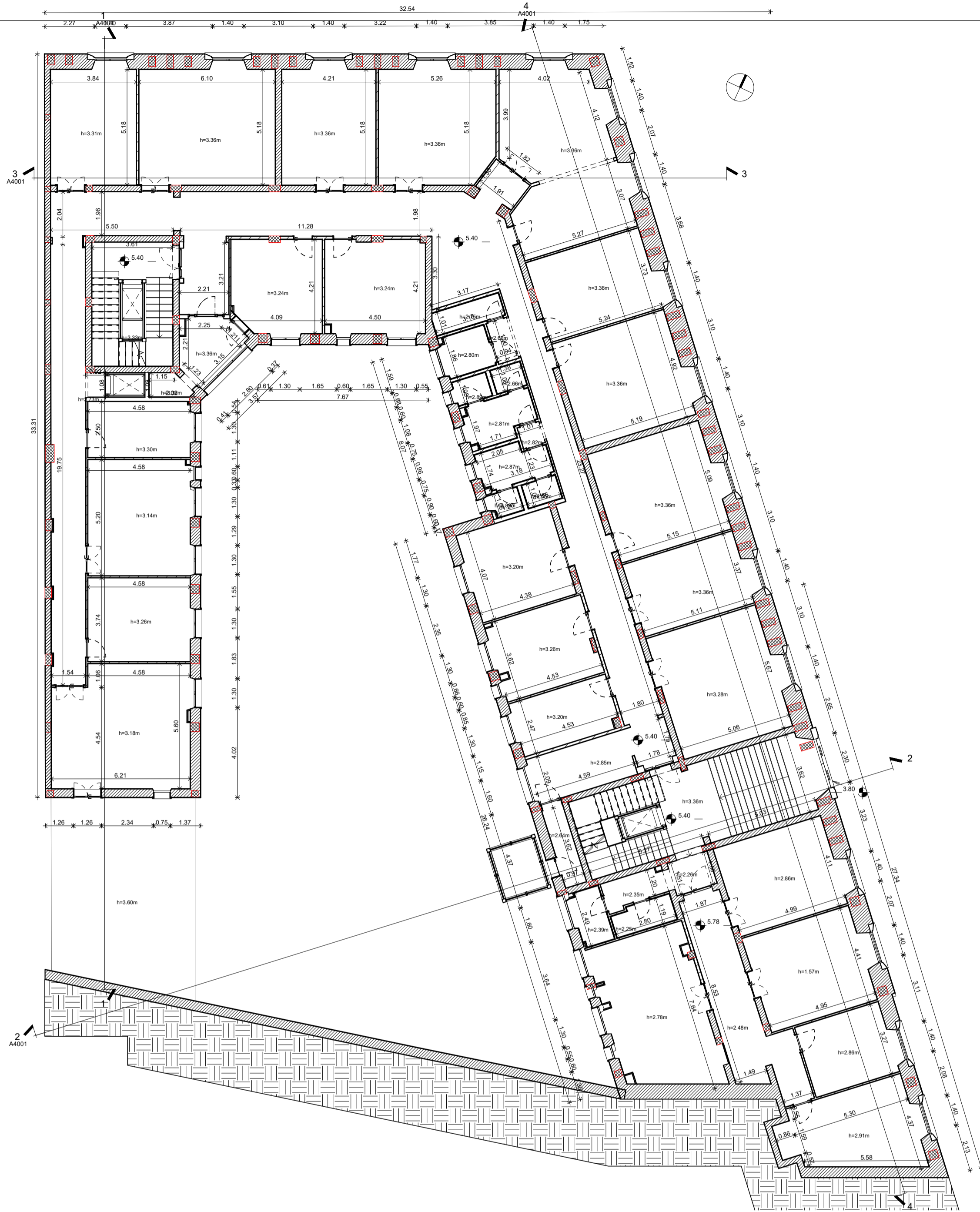
A_01_Dimensionale Scala 1:100
