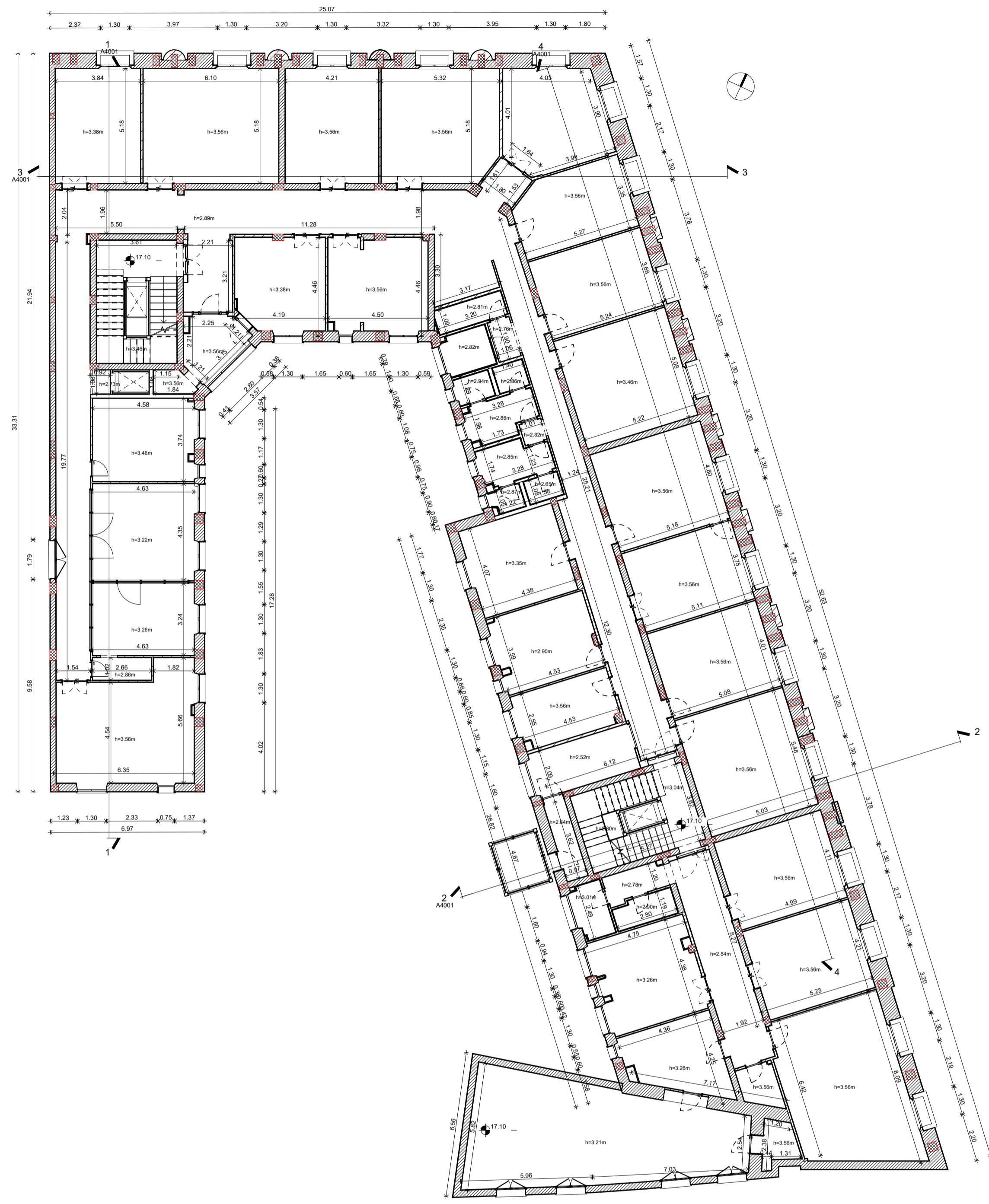
A_04_Dimensionale Scala 1:100
