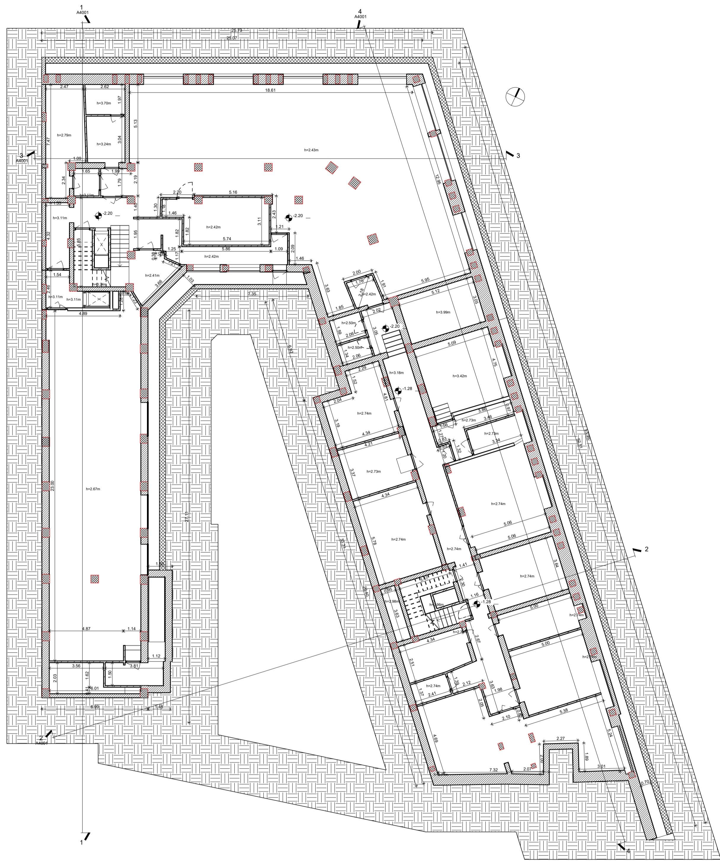
A_LG1_DimensionaleScale 1:100
