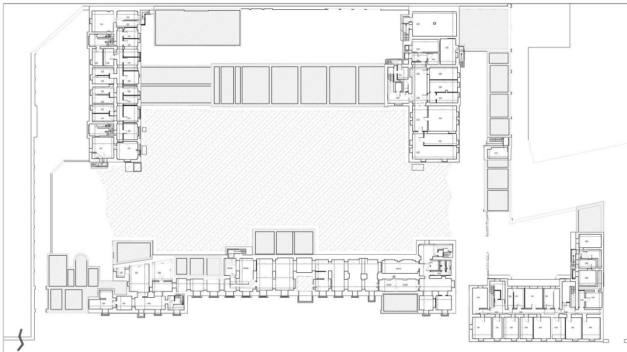
Figura 1: Planimetria piano interrato
