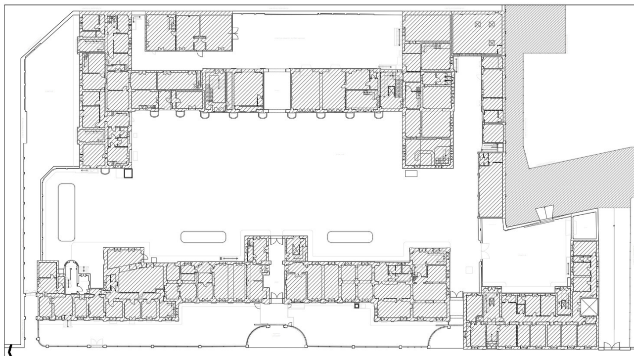
Figura 2: Planimetria piano terra
