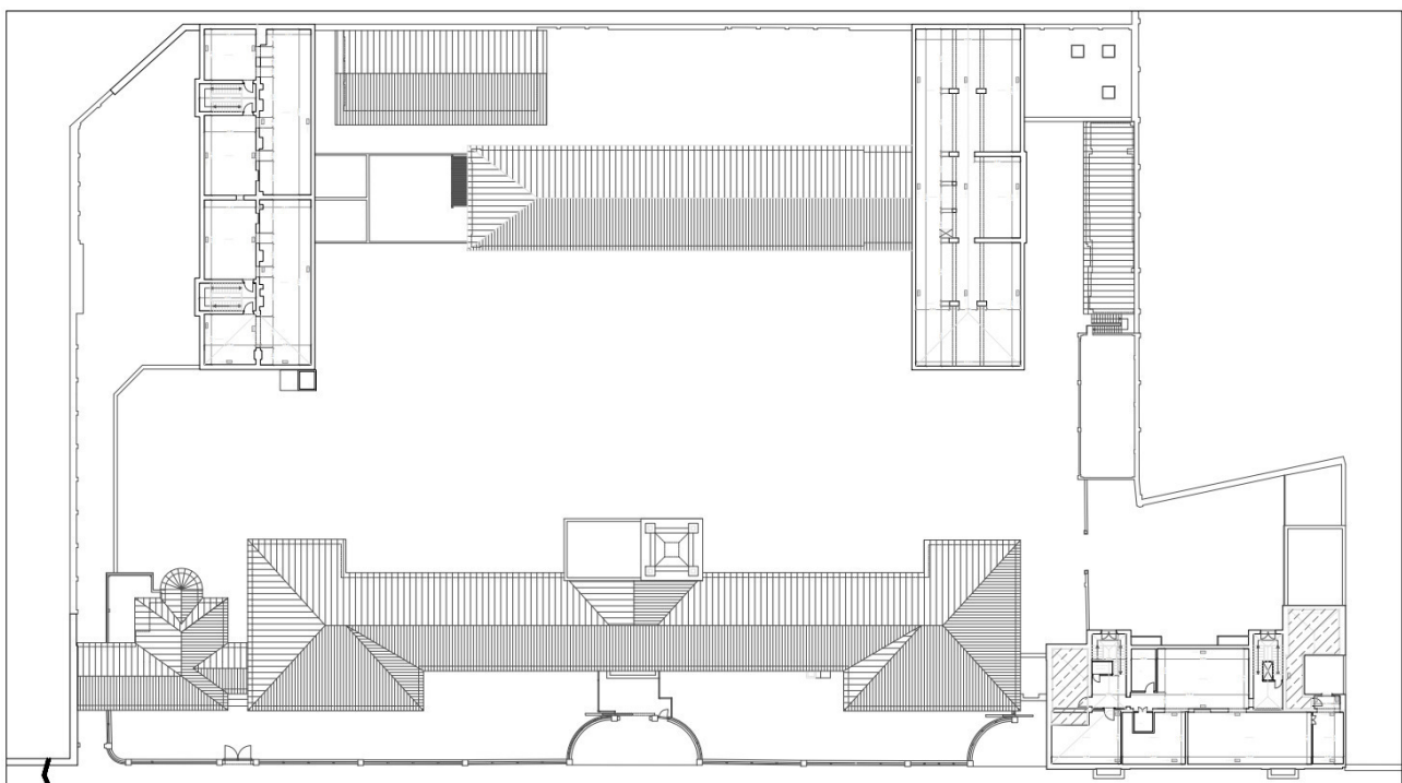
Figura 8: Planimetria sottotetti
