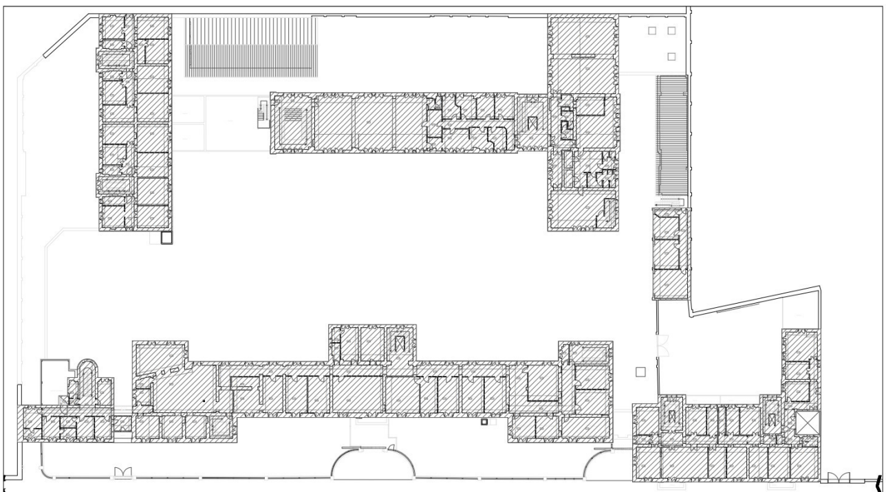
Figura 4: Planimetria primo piano
