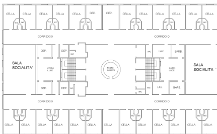
CORPO N PIANO QUARTO H=3.00
