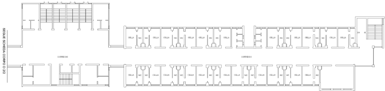
CORPO D PIANO TERZO SCHEDA 2/2 H 3.00m
