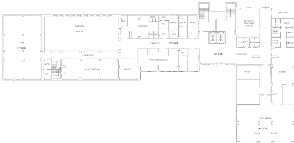
CORPO A PIANO TERRA
