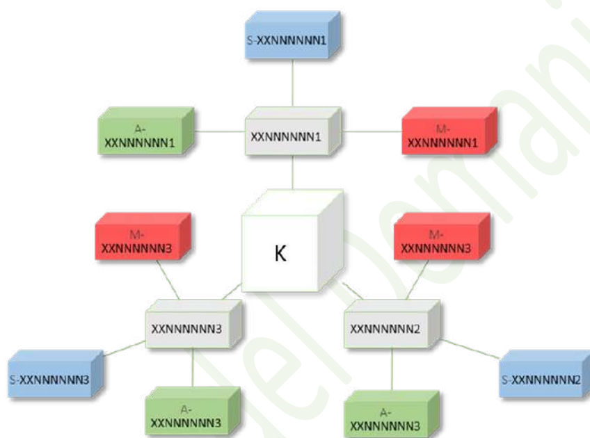
Figura 6 - Esempio Modello federato Complessivo/di Fabbriato (K)
