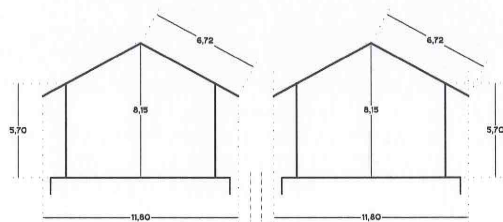
Sezione AA' - scala 1:200
