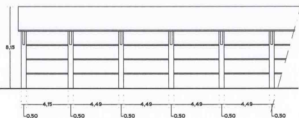
Prospetto Longitudinale "P"
