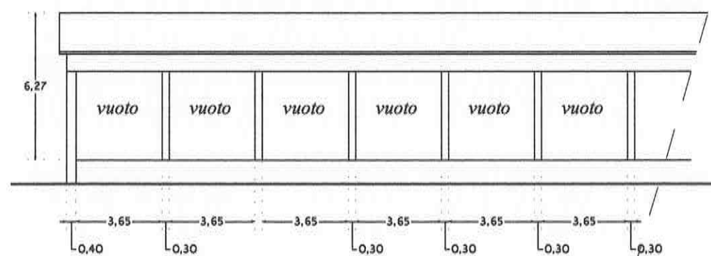
Prospetto Longitudinale "P"
