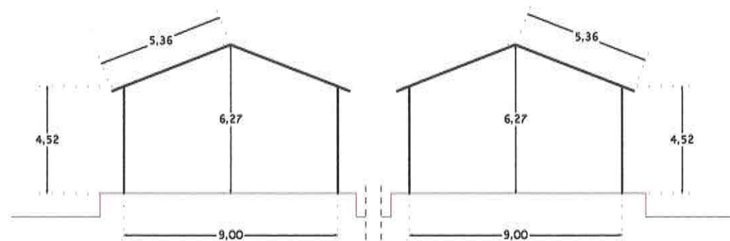
Sezione AA' - scala 1:200
